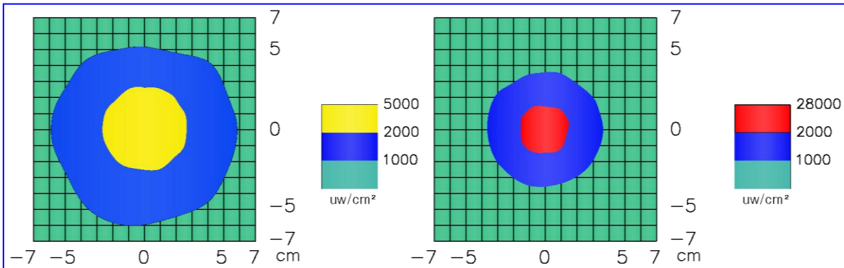
UV 辐照度强度分布图 (380mm)
