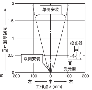
带圆形狭缝透光罩(φ 1mm)时的平行移动特性
