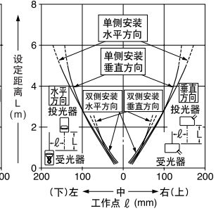
带方形狭缝透光罩的平行移动特性 (2 × 6mm)
