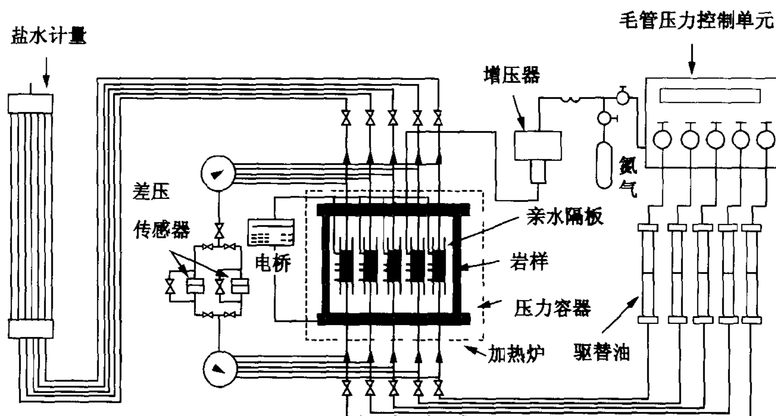
图 1 半渗透隔板驱替装置示意图
