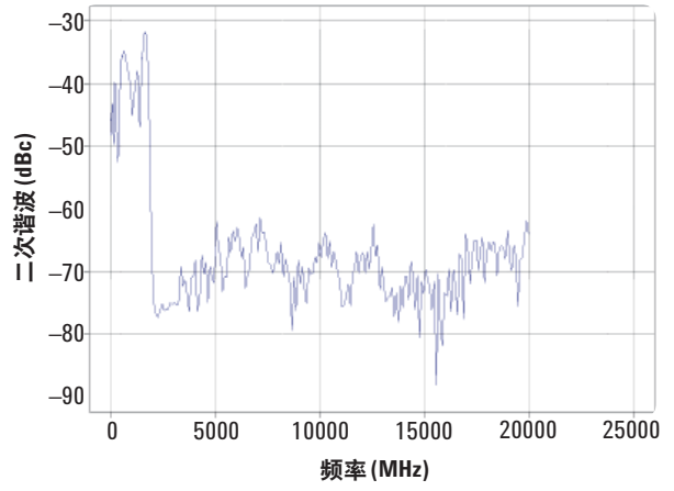
选件 520 在 +20 dBm 时的谐波 (测量值)
