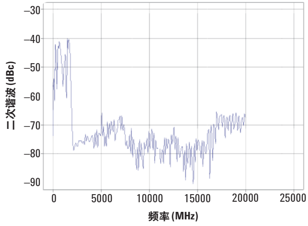
选件 520 在 +10 dBm 时的谐波 (测量值)
