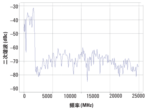
选件 540 在 +20 dBm 时的谐波 (测量值)
