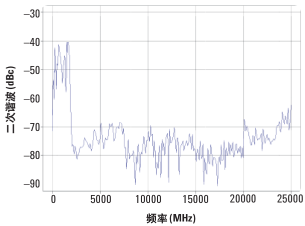
选件 540 在 +10 dBm 时的谐波 (测量值)
