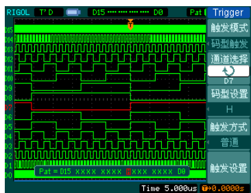
码型触发
