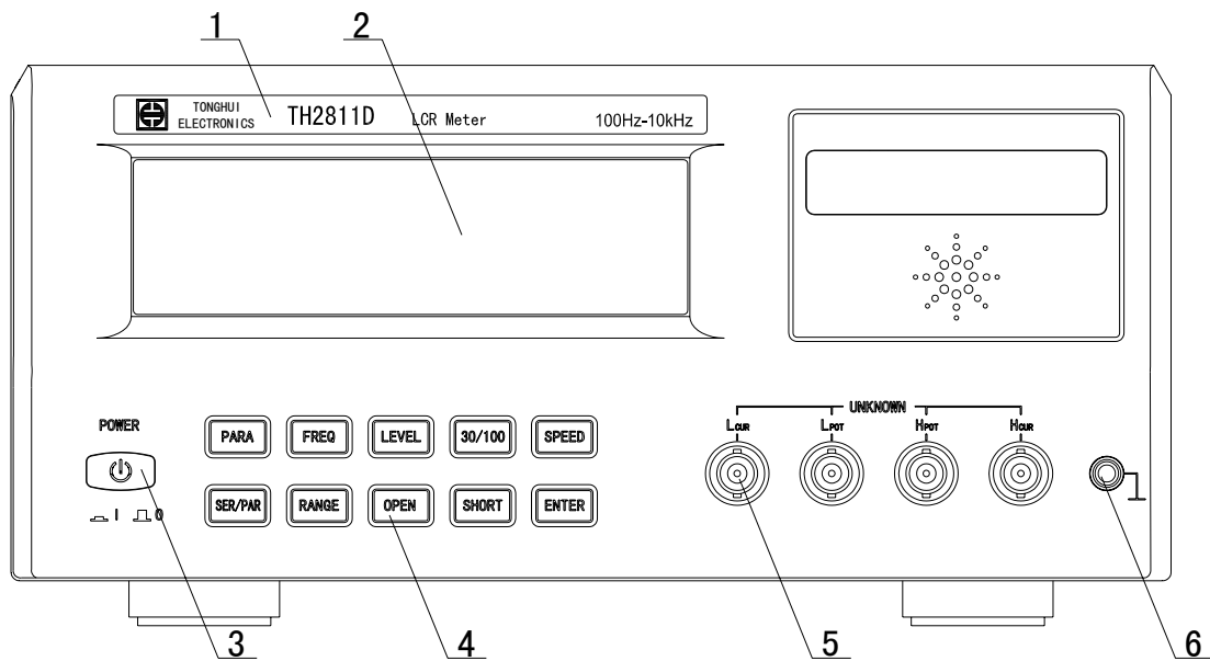
图 2-1. 前面板
