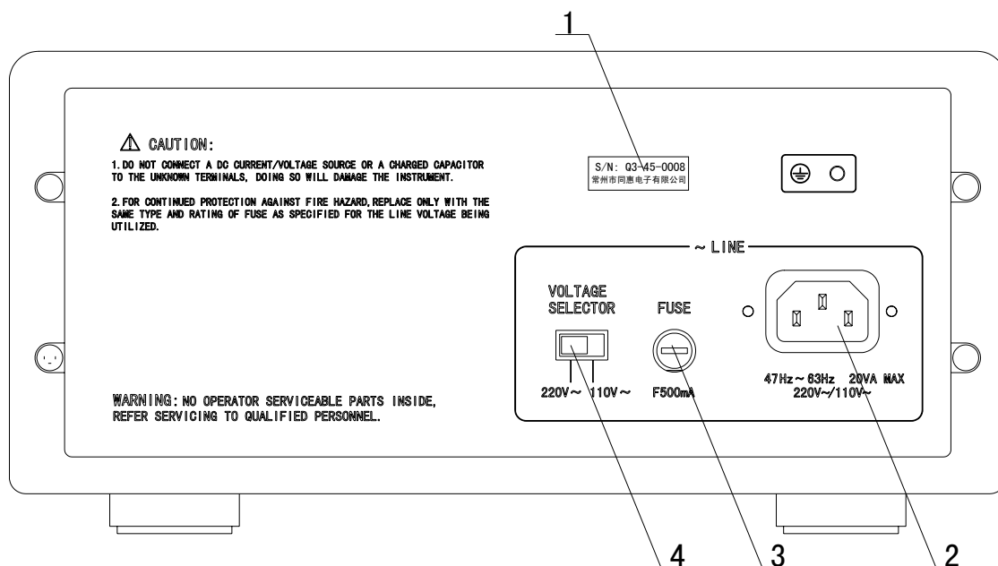
图 2-2. 后面板
