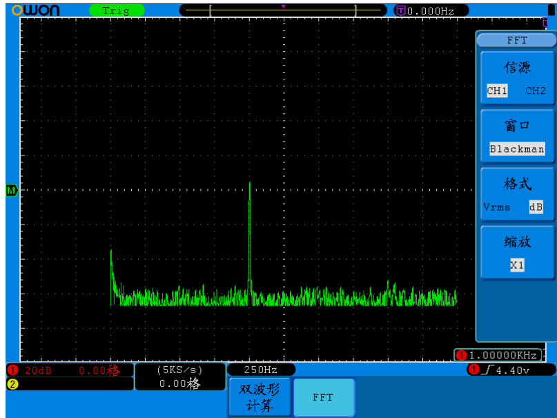
图 5-10: BLACKMAN 窗
