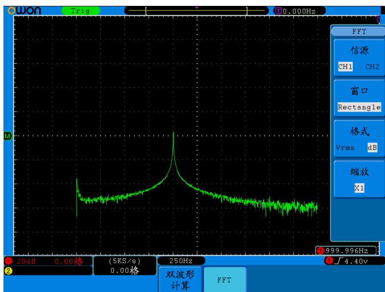
图 5-12: RECTANGLE 窗
