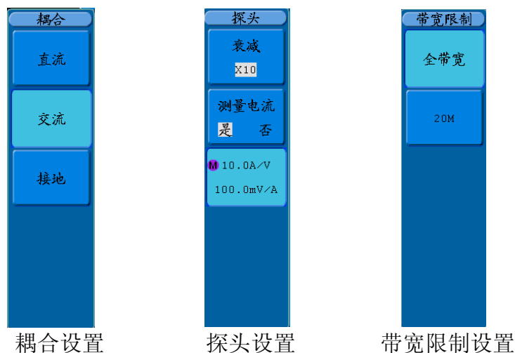
图 5-1：通道设置菜单（SDS6062(V)无“带宽限制”菜单）
