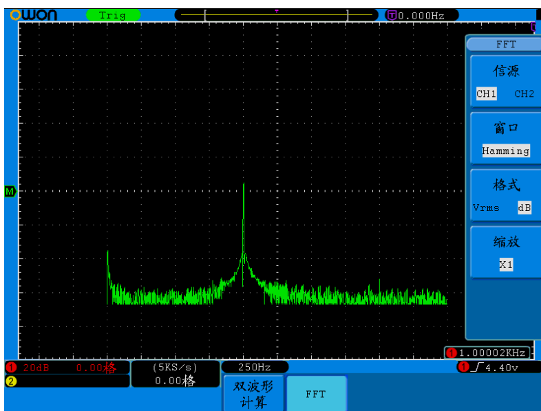
图 5-13: HAMMING 窗
