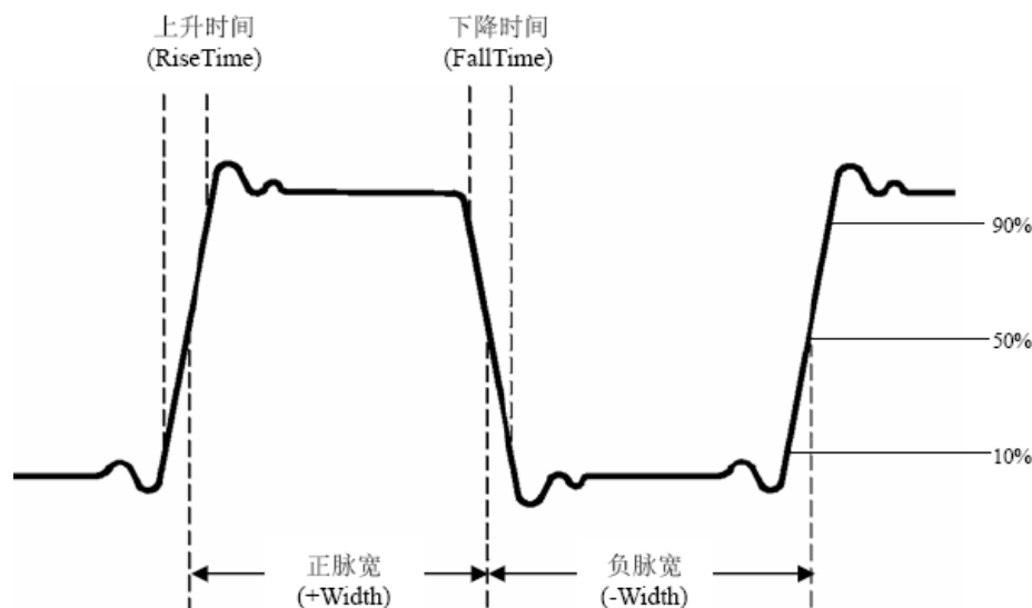
图 5-59: 时间参数定义示意
