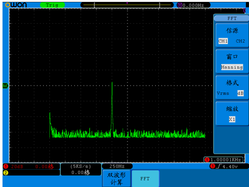
图 5-11: HANNING 窗
