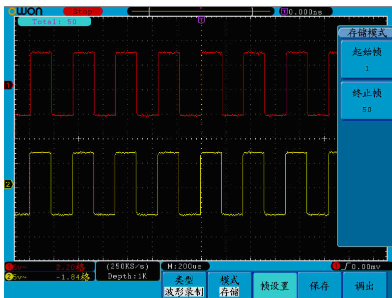
图 5-41：波形存储
