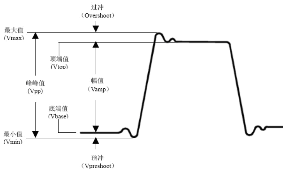
图 5-58: 电压参数定义示意 (顶端平整有脉冲信号)
