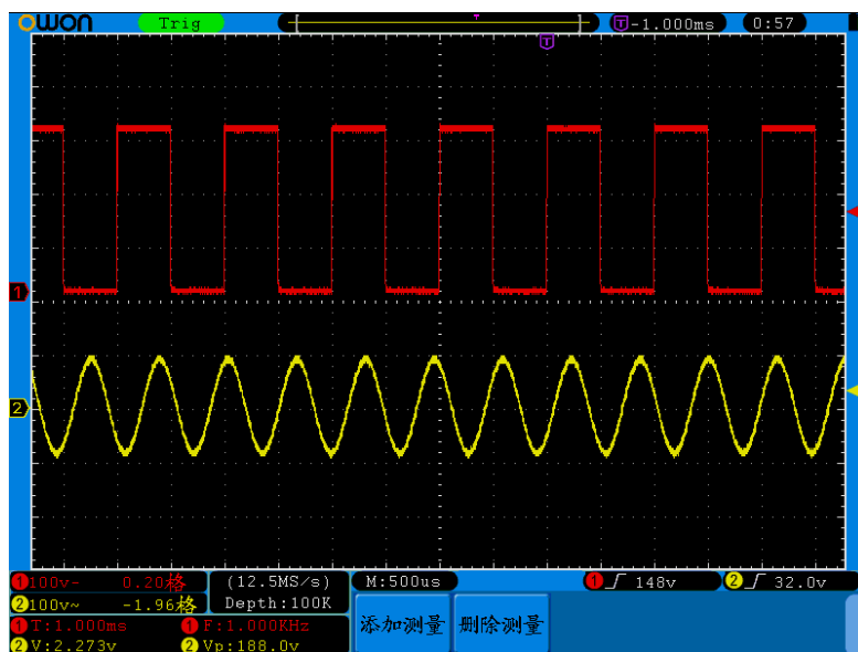
图 5-57: 自动测量
