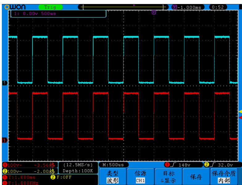
图 5-37：波形储存
