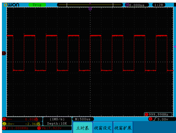
图 5-16: 主时基
