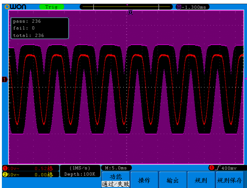
图 5-47: 通过/失败检测
