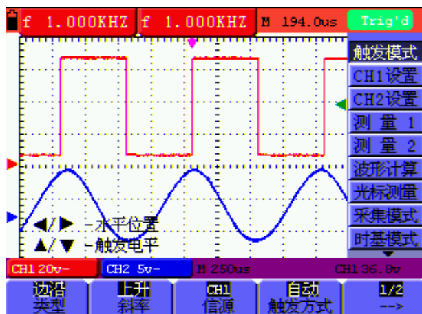
图 39：边沿触发
