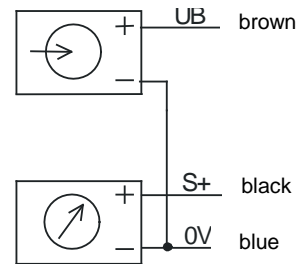
Cable outlet
