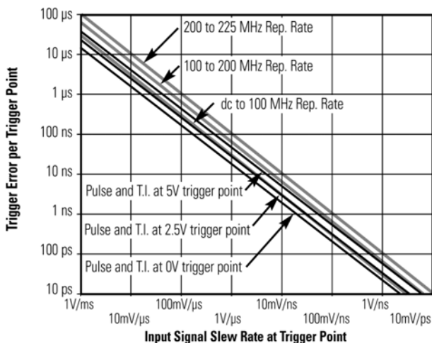
图 6: 触发电平定时误差 (电平设置误差和输入滞后)
