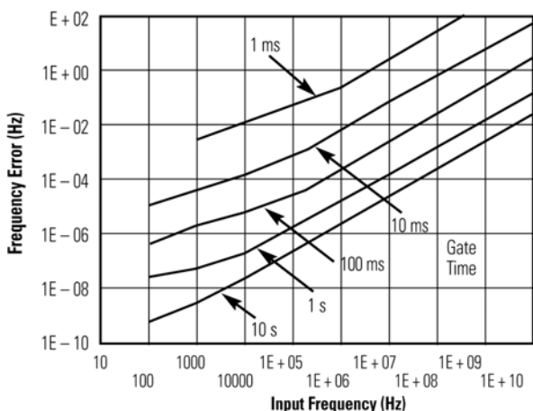
图 5: Agilent 53132A —最坏情况 RMS 分辨率 7 (时间或位数同步)
