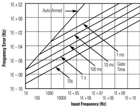
图 4: Agilent 53132A —最坏情况 RMS 分辨率 7 (自动或外部同步)
