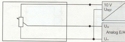
电位差计接线示意图
