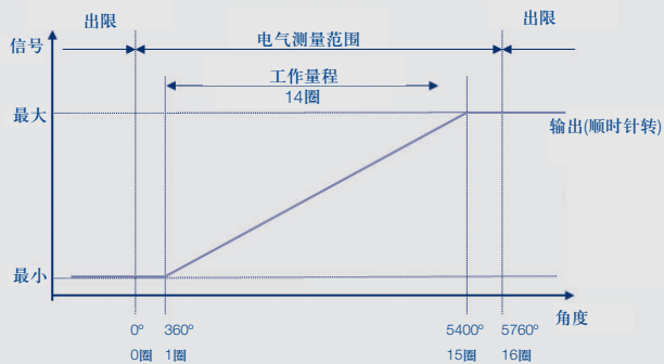
工作量程14圈输出信号
