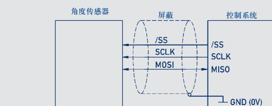
SPI输出接线图
