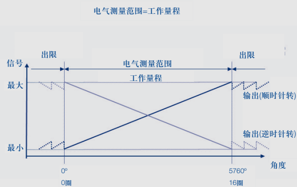
工作量程16圈输出信号
