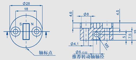
磁块 Z-RFC-P08（辅件）
