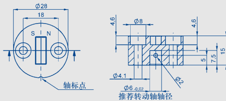
磁块 Z-RFC-P02（辅件）
