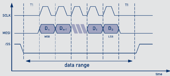
接口定义（SPI输出）
