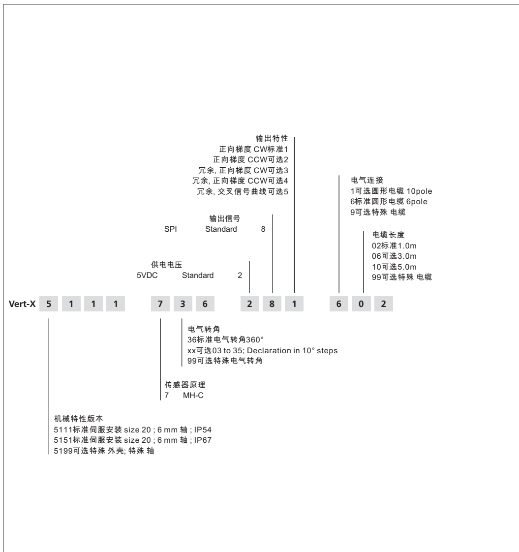
Vert-X 51 - 5V / SPI 订购代码
