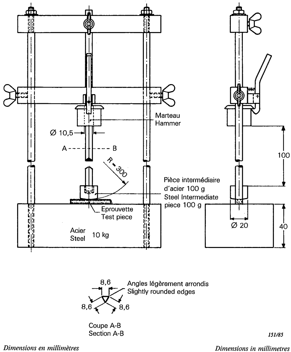
FIG. 2.— Appareil d'essai de choc. Impact test apparatus.
