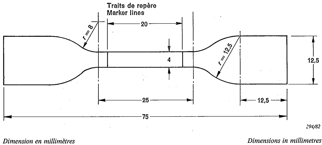
FIG. 3.— Epreuve en forme d'haltère. Dumb-bell test piece.
