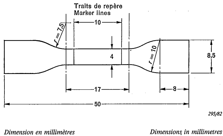
FIG. 4.— Petite éprouvette en forme d'haltère. Small dumb-bell test piece.
