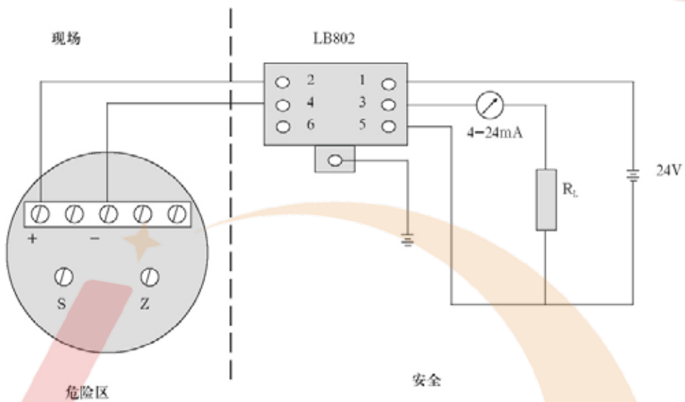
防爆型变送器与安全栅接线图
