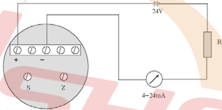
普通型变送器接线图
