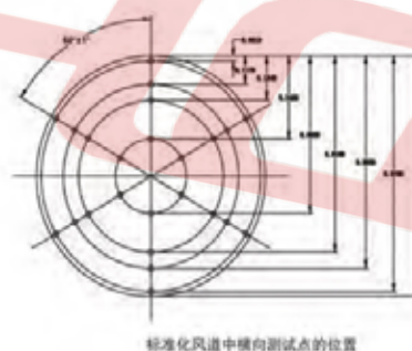
标准化风道中横向测试点的位置
