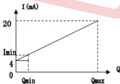
4~20mA电流输出特性
