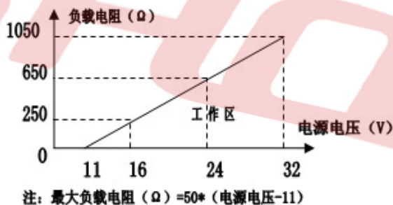
4~20mA电流输出负载特性
