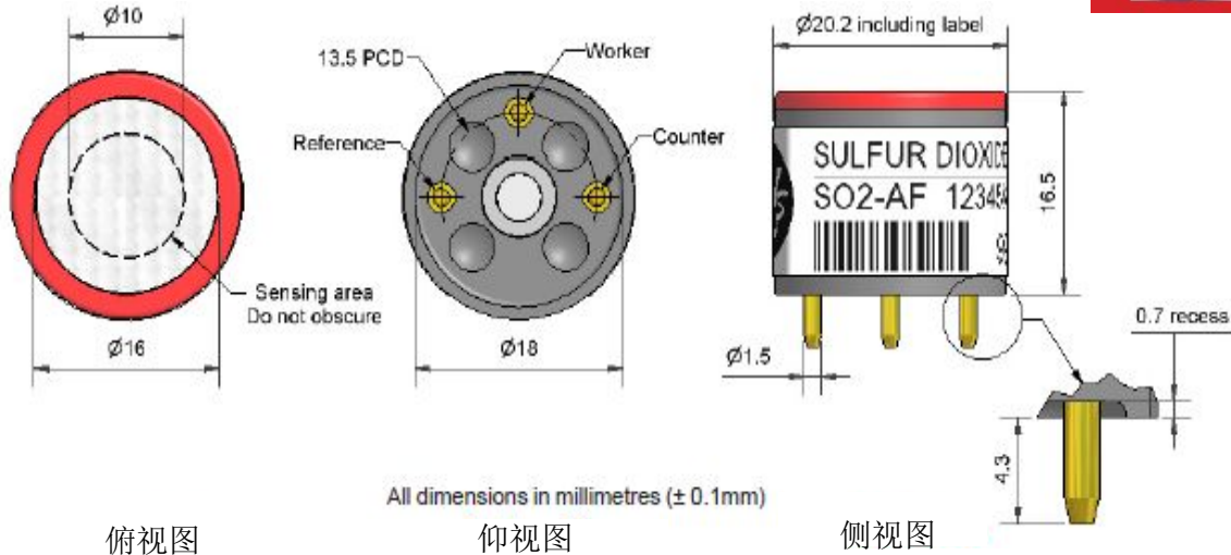
图1 SO2-AF示意图
