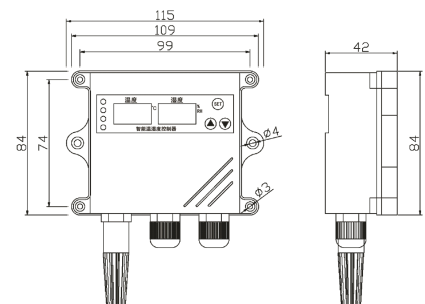
外形尺寸图
