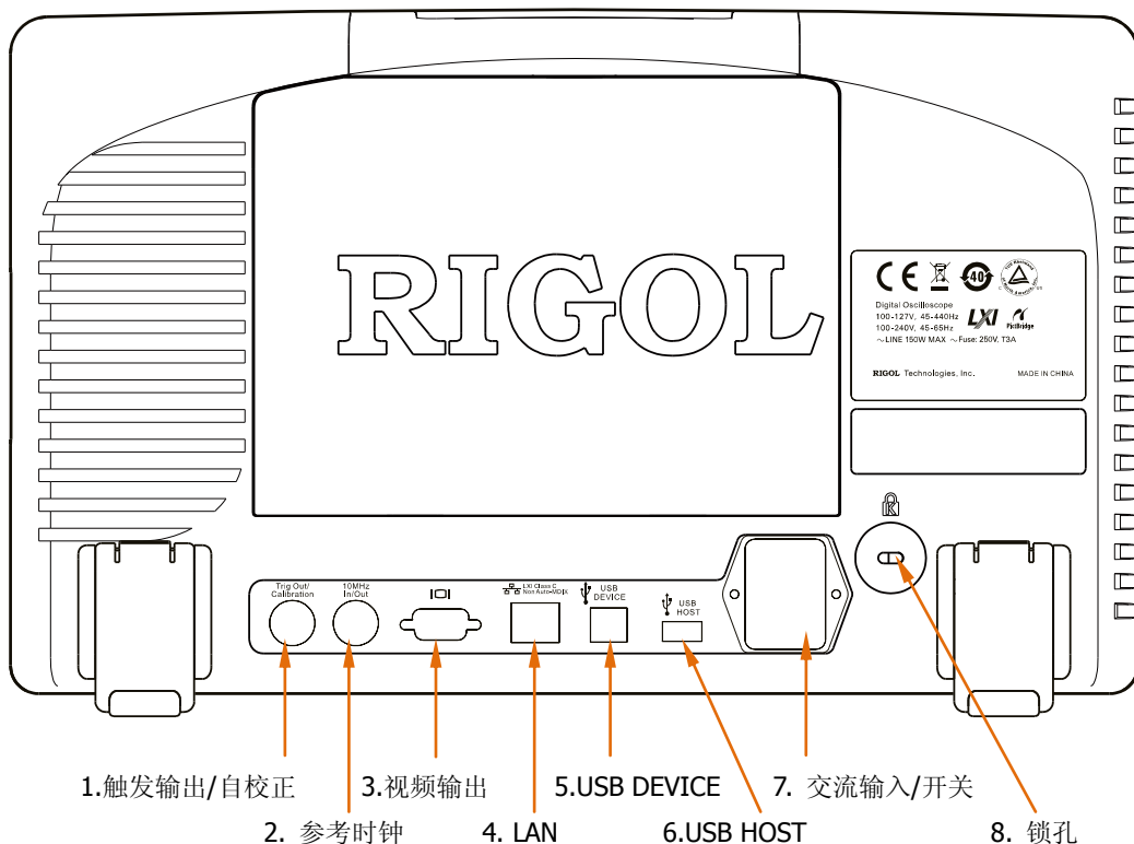
图 1-12 后面板总览
