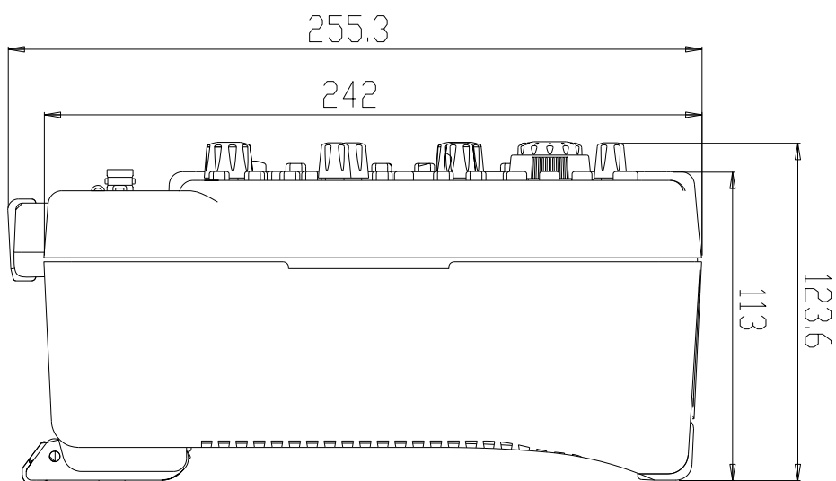
图 1-2 侧视图
