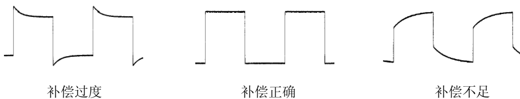
图 1-10 探头补偿
