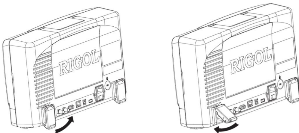
图 1-4 调节支撑脚
