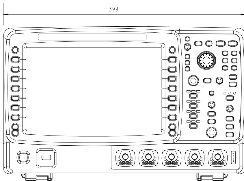
图 1-1 正视图
