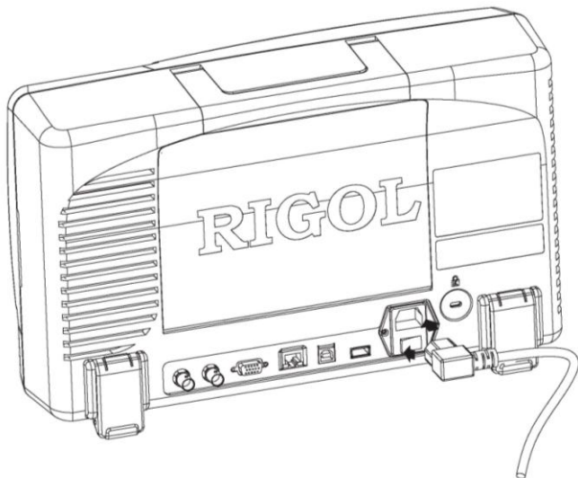
图 1-5 连接电源
