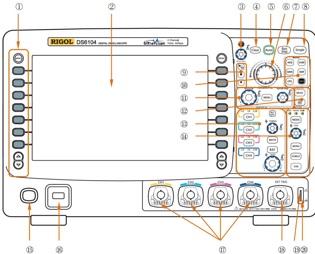
图 1-11 前面板总览
