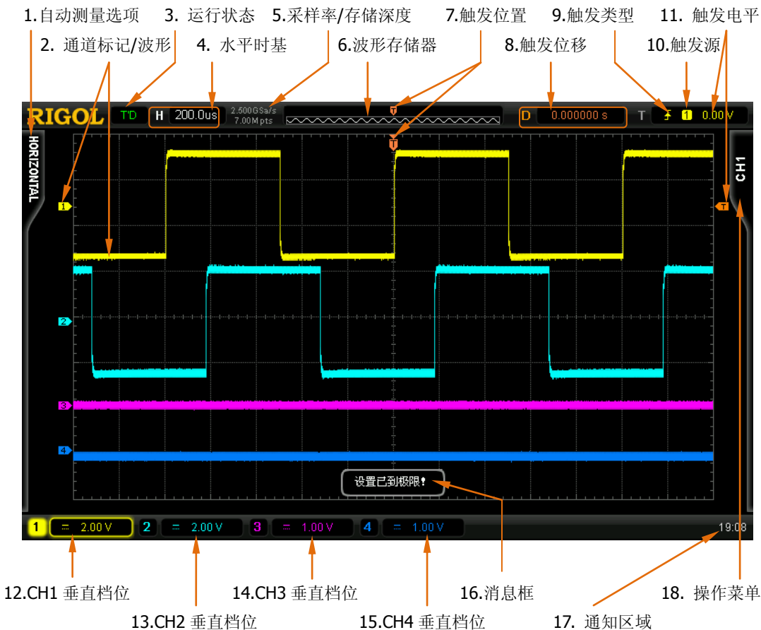
图 1-13 用户界面
