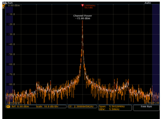
自动测量信道功率
