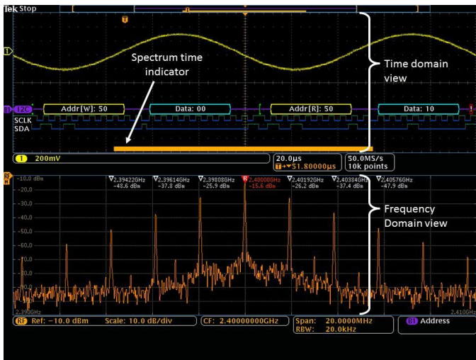
MDO4000C 系列显示屏上半部分显示模拟通道和数字通道的时域视图，下半部分显示频谱分析仪通道的频域视图。橙色短条（即频谱时间）显示用于计算射频频谱的时间周期。
