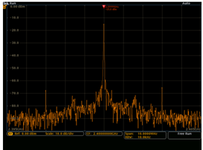
MDO4000C 频域显示。
