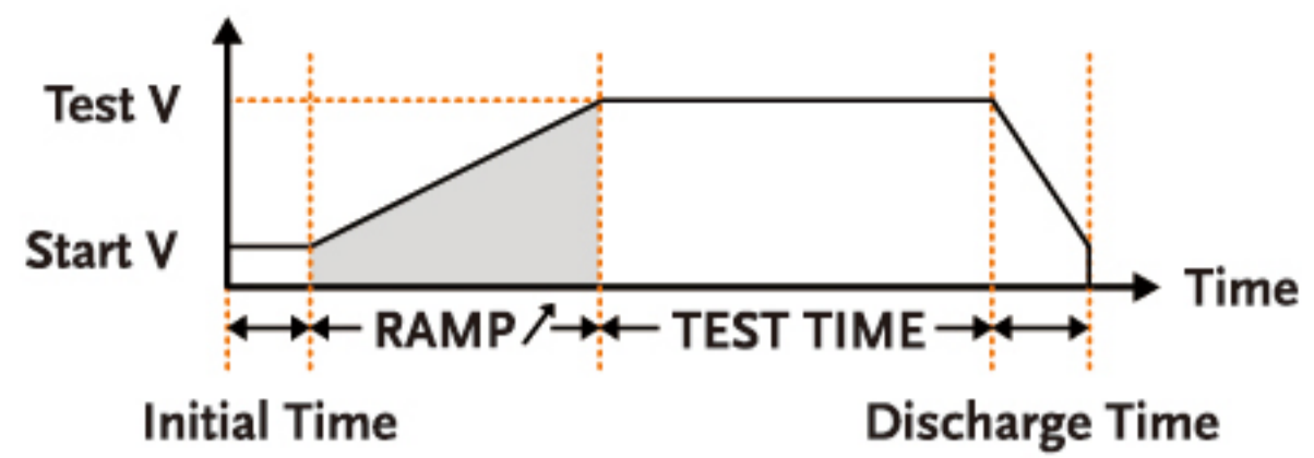
一个测试周期内输出电压可调
