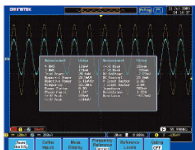
电源质量
