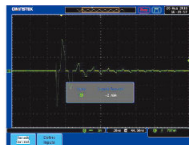
浪涌电流
