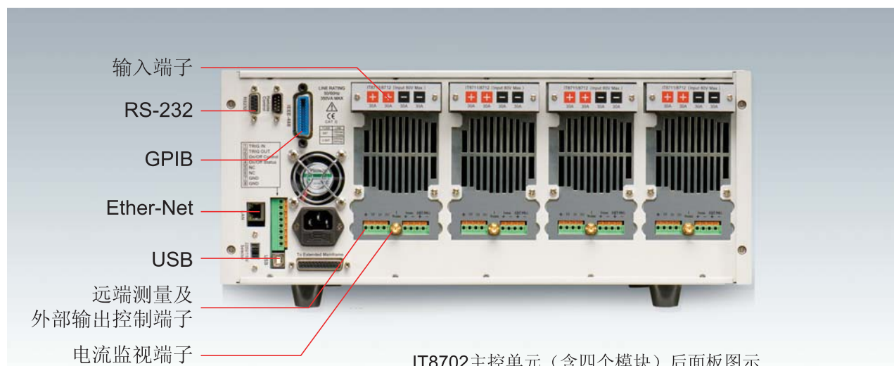
IT8702主控单元（含四个模块）后面板图示
