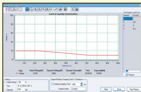
PV8500 电池放电测试界面
