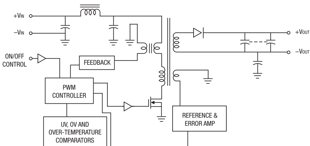
ULE-12/4.2-D48N
