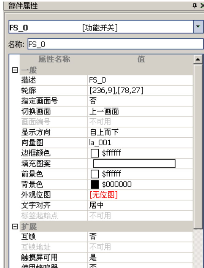
图 13-8 功能开关部件属性表
