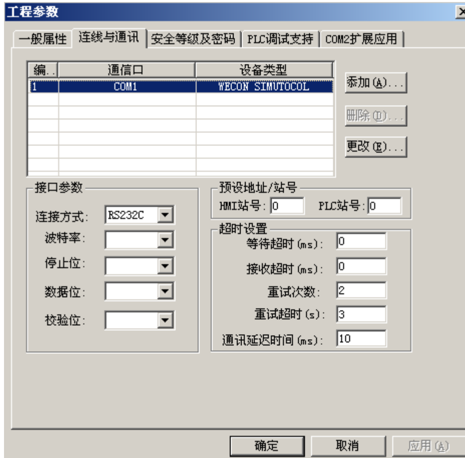
图 7-2 通讯参数设置
