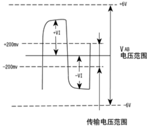
图 23-3 传输电压范围
