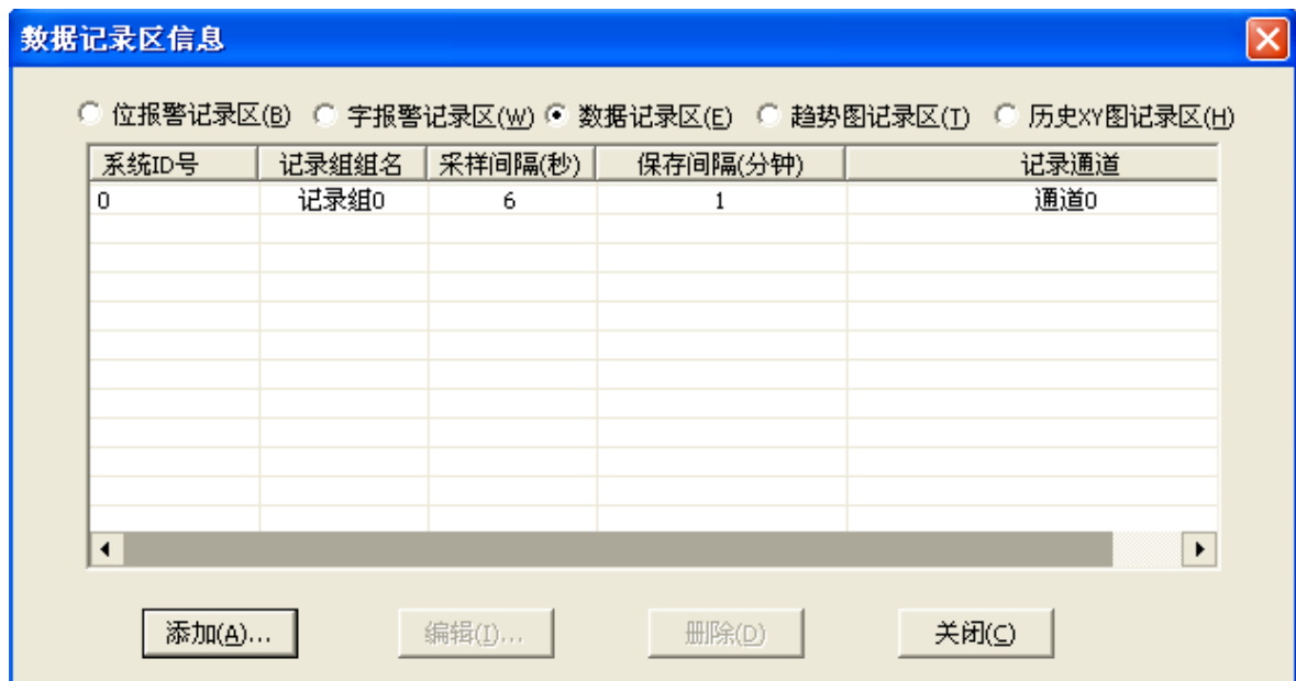
图 26-2 数据记录区
