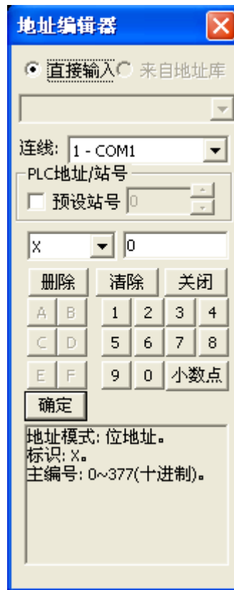
图 9-1 地址编辑器
