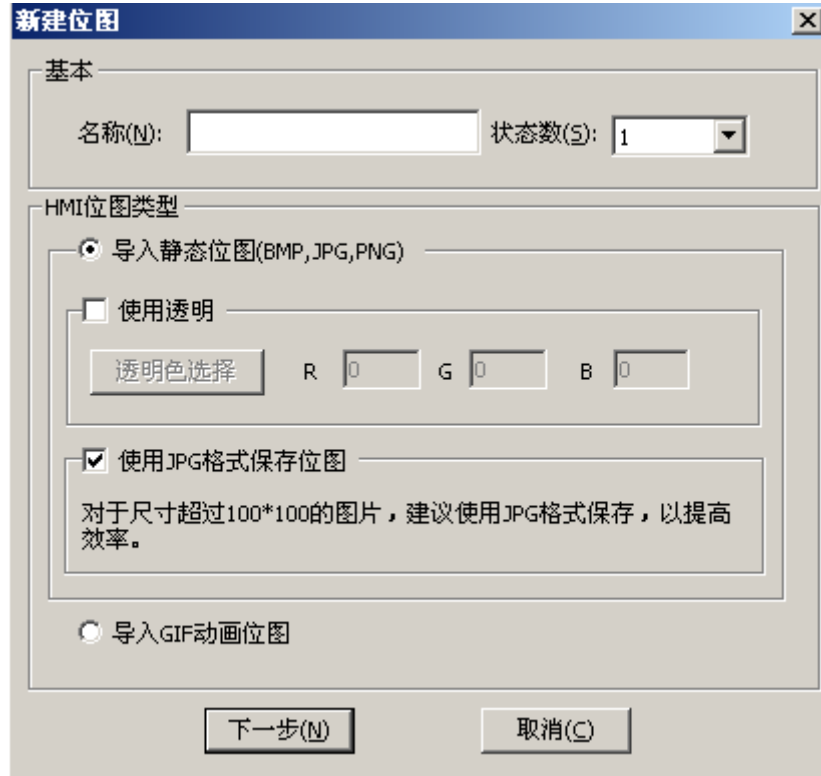
图 8-2 新建位图
