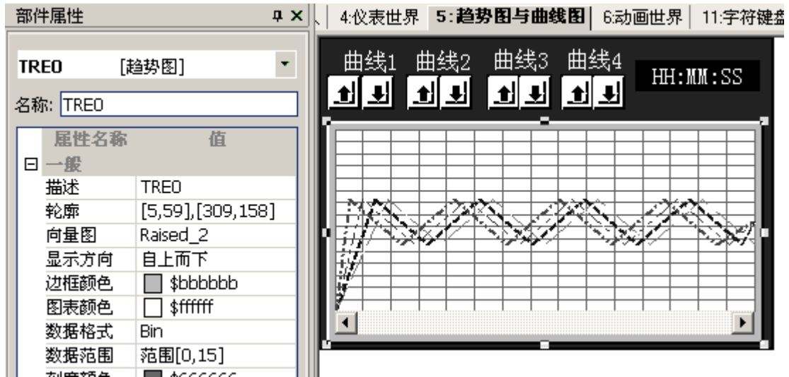
图 13-25 趋势图示例
