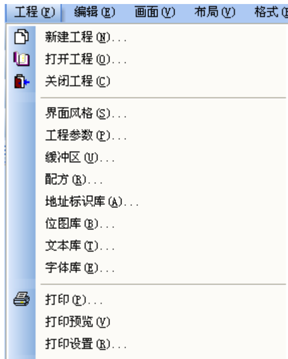
图 3-2 工程菜单
