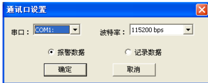
图 26-7 通讯口设置
