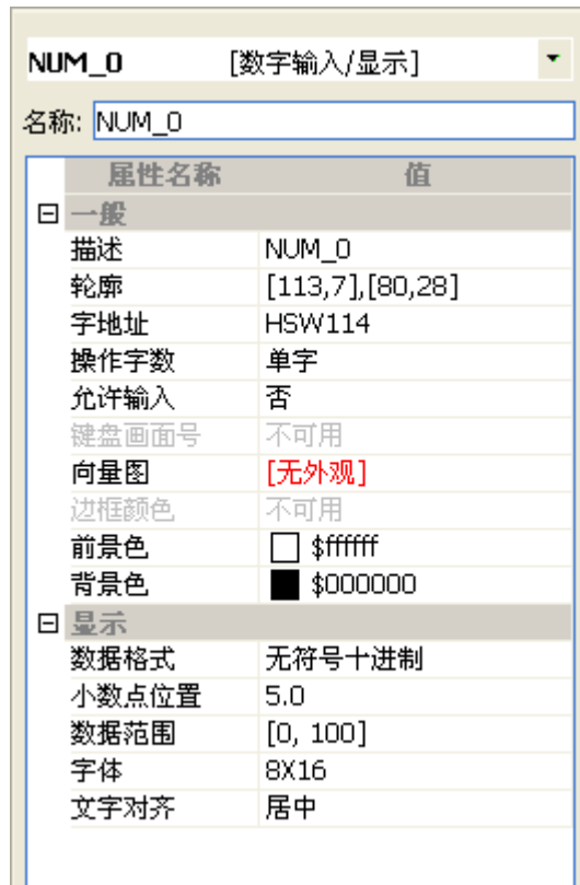
图 16.3 显示当前安全等级
