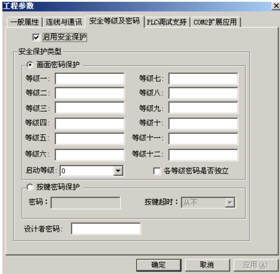
图 7-3 安全等级设置
