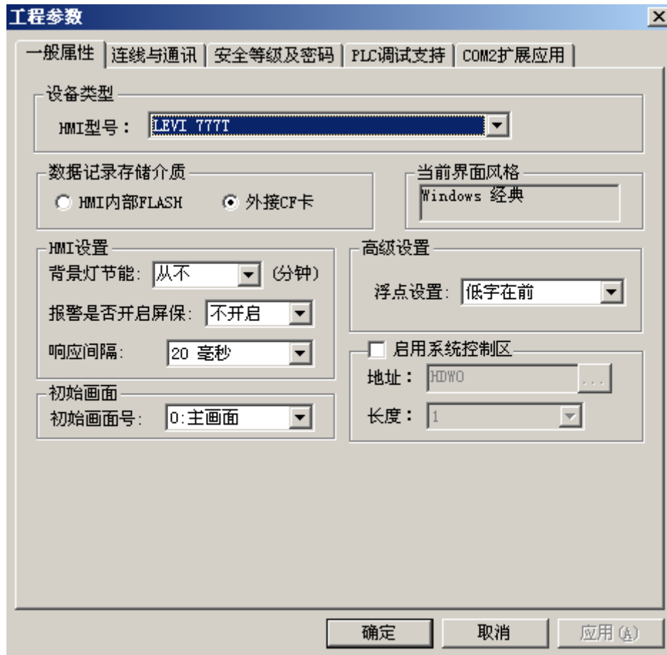
图 7-1 一般属性
