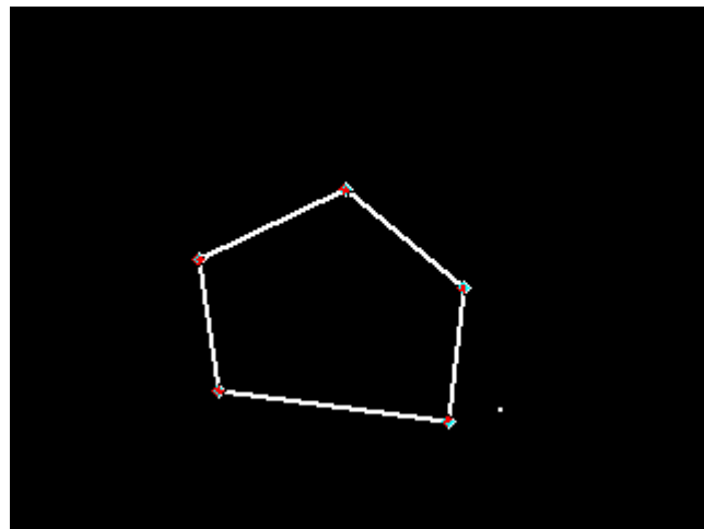
图 10-3 选中多边形
