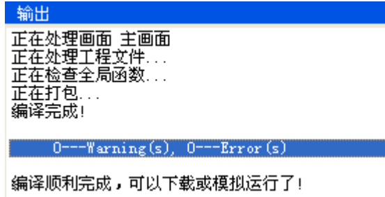
图 5-15 输出窗口
