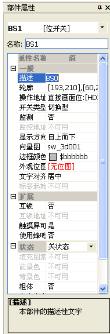
图 3-11 部件属性框
