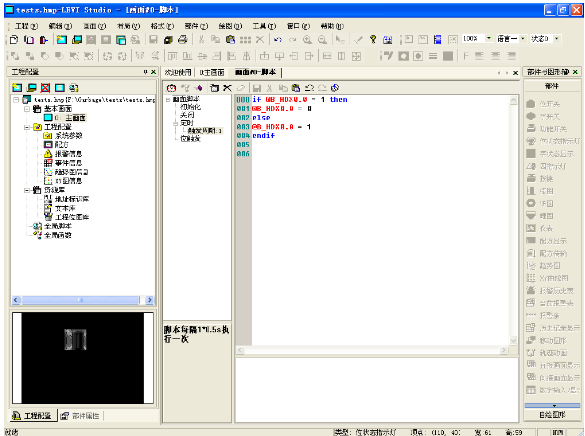
图 17-5 脚本编辑器
