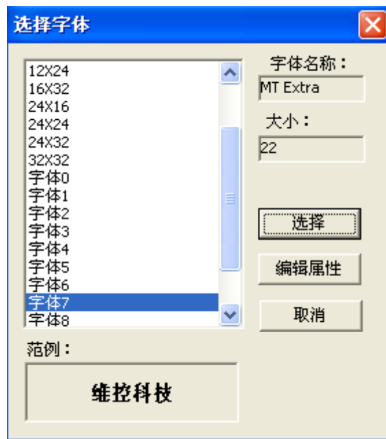
图 25-5 选择字体
