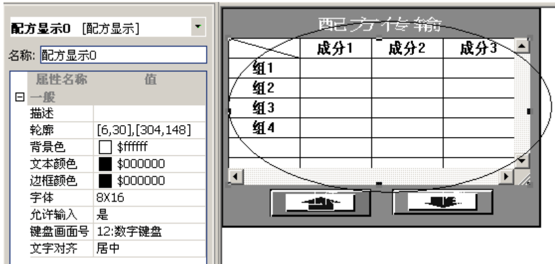
图 13-22 配方示例
