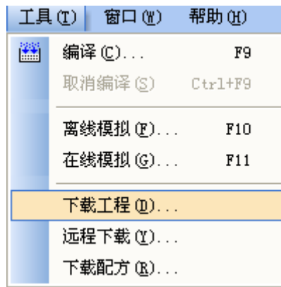
图 19-1 下载工程
