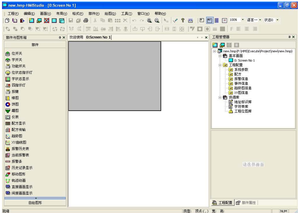
图 5-5 窗口布局
