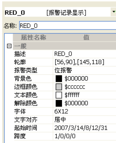
图 13-50 报警记录显示示例
