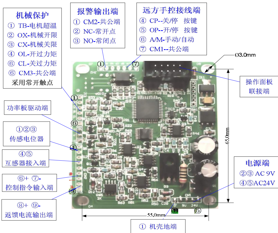
远方控制接线图
