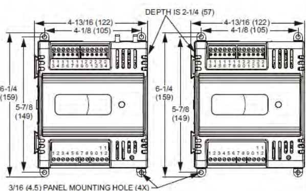
图2. 面板安装-控制器尺寸适用于PUB1012S, PUB4024S和PVB4024NS (图为PUB4024S和PVB4024NS)
