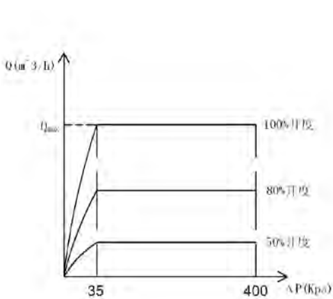
压差流量特性
