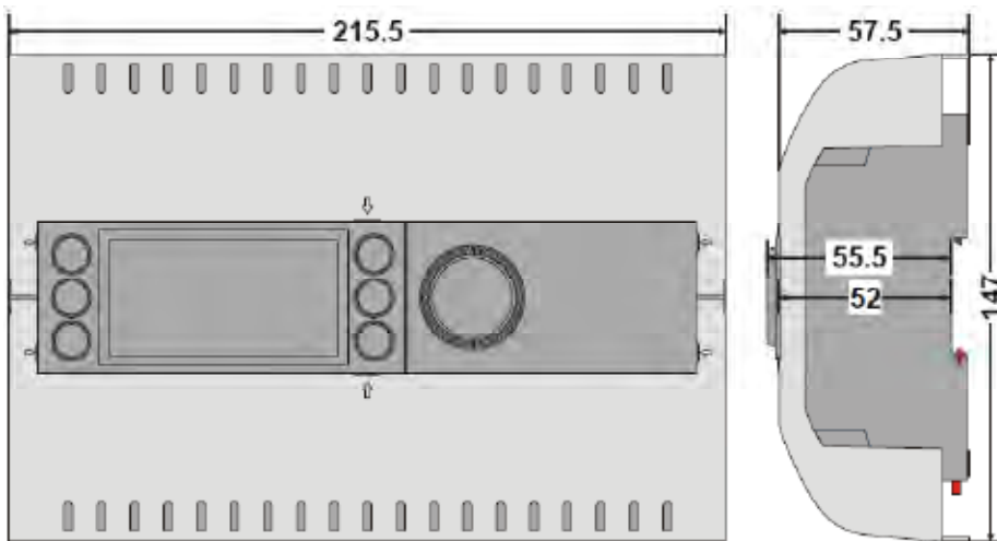
图10. MVC 控制器 (MVC-80M-CPSW1A, 端子盖), 外形尺寸 (mm)
