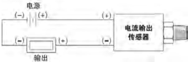
电流输出型电气接线图：
