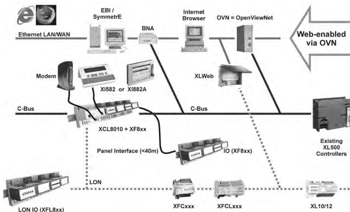
图1.系统结构图
