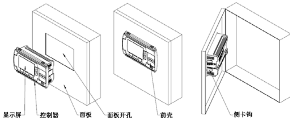
图2 面板安装
