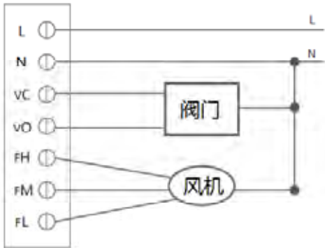
图3. VC6013/VN6013 系列阀门接线示意图
