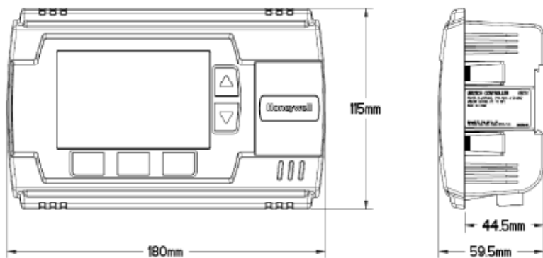
图1 产品尺寸
