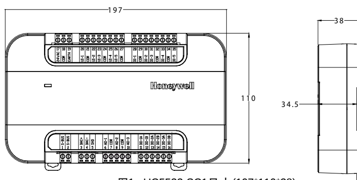
图1 . UC5533-SC1尺寸 (197*110*38)
