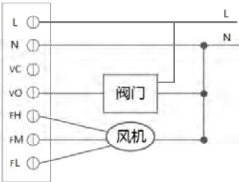
图2. VC4013/VN4013/VS4016 系列阀门接线示意图
