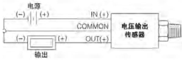
电压输出型电气接线图：
