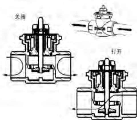
图1: 2通VN系列1/2"和3/4"阀门的液体流向
