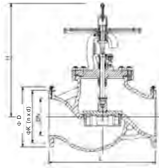
图3 Kombi-SV DN250-DN350
