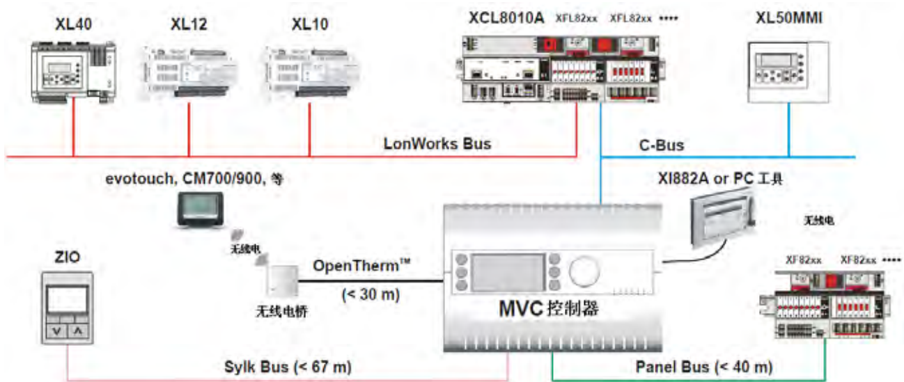
图1. MVC 控制器与Excel 5000系统结构
