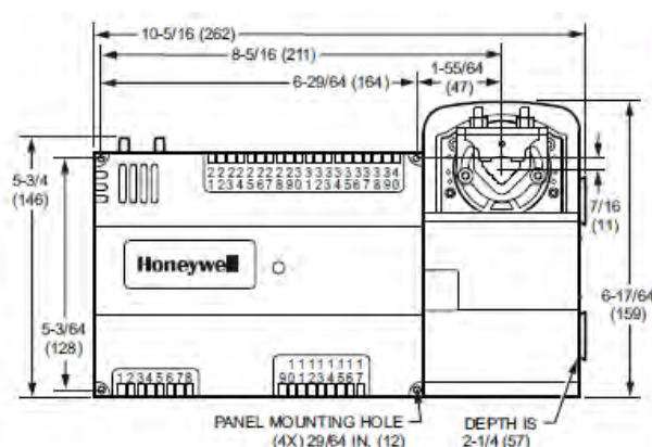
图3. 面板安装尺寸适用于PVB6436AS
