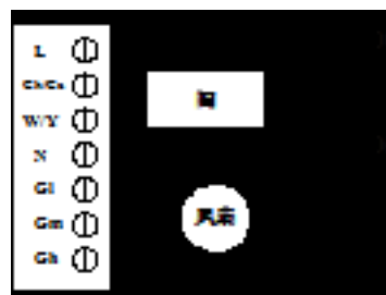
VC6013 阀接线图
