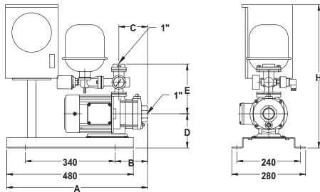
● 圖3. TPH4T2KICV / TPH4T3KICV
