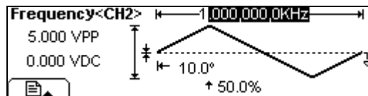
图 3-24 复制后通道 2 波形参数
