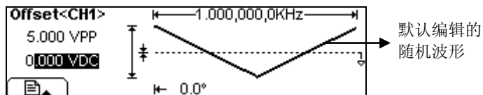
图 2-32 图形显示模式下的波形
