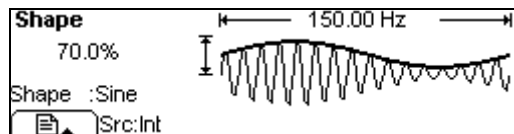
图 3-9 输出 AM 调制波形
