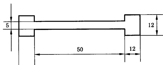
图 3 哑铃试样
