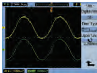
通道 1 波形 (黄色) 显示未经滤波的输入信号，通道 2 波形 (绿色) 显示同一输入信号经过低通滤波后的结果
