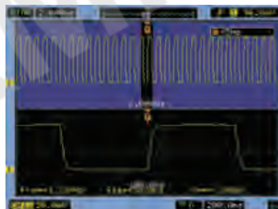
可在查看一段较长时间记录的同时, 在缩放窗口中观察信号的细节
