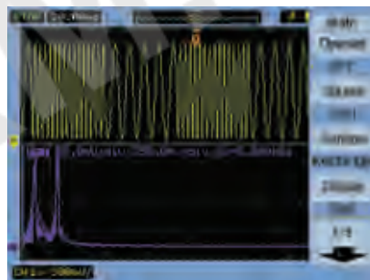
内置 FFT 函数可快速对时域信号实施频谱分析
