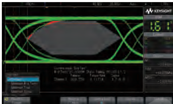
模板测试在短短2分钟内测试了超过2700万个波形
