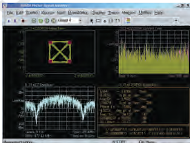
使用矢量信号分析软件查看FFT频谱分析
