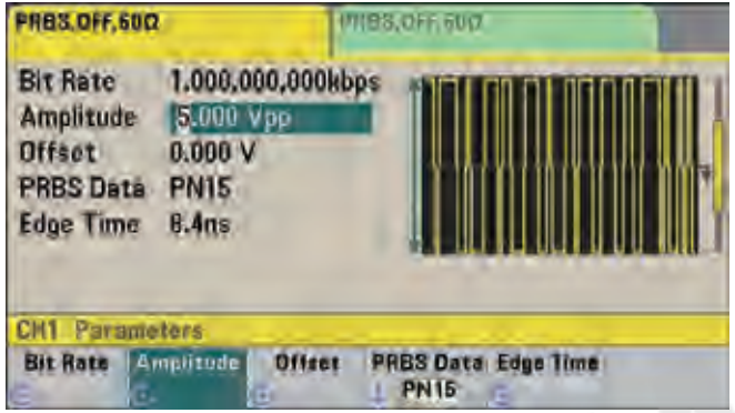
33622A 显示输出: 双通道追踪用于生成差分输出
