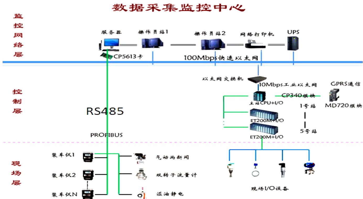
罐区PLC监控及全自动装车系统图
