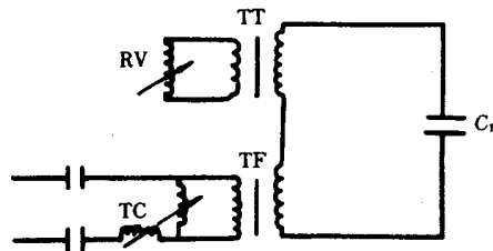
图 A1 工频串联谐振试验回路 TC—单相调压器;TF—馈电变压器;RV—可调电抗器; TT—升压变压器; C_p —试样
