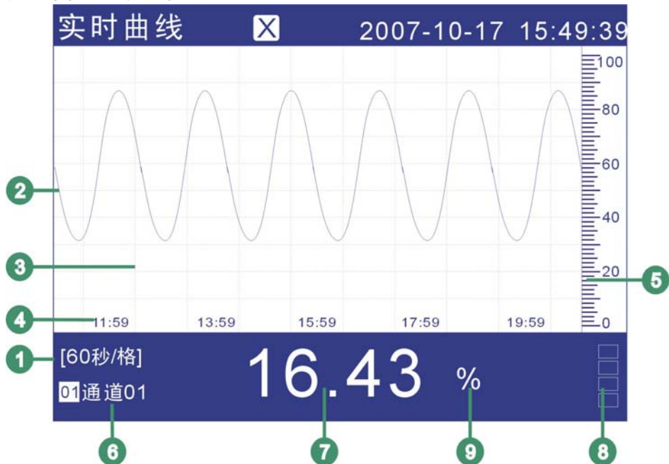
实时曲线显示（横向）
