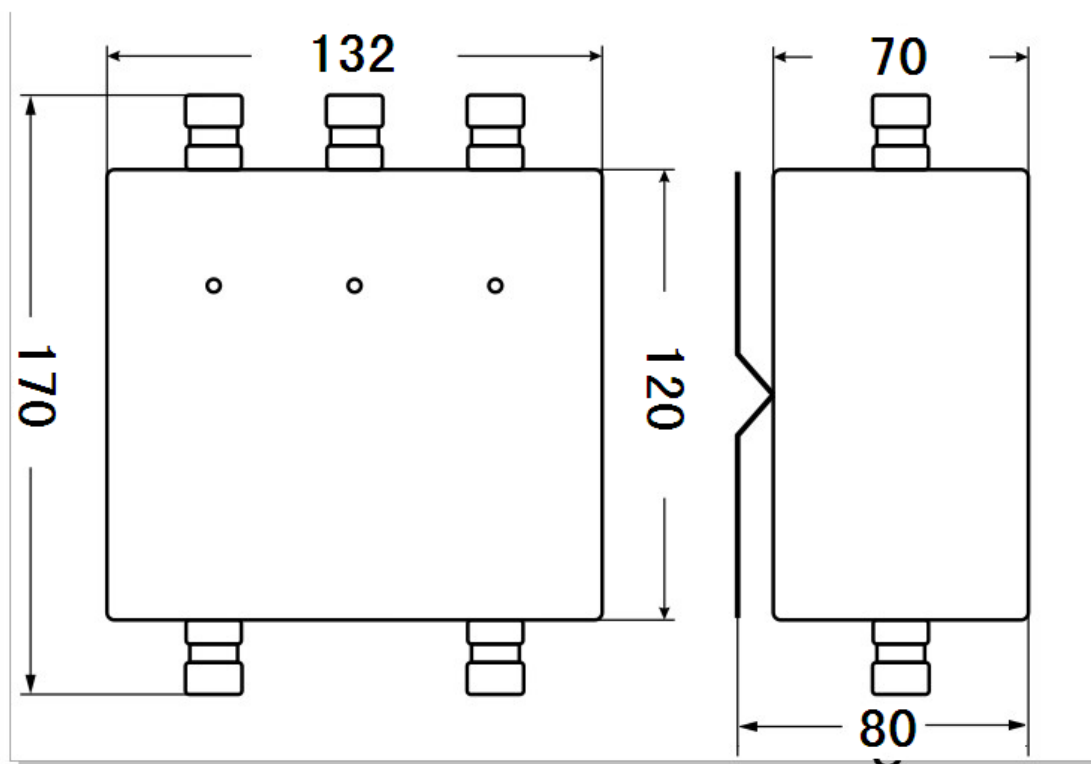
KYXBQ-1000-3尺寸图
