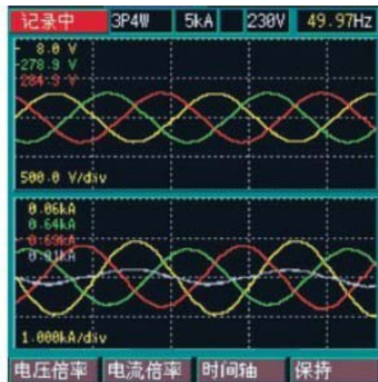
谐波治理后测试数据
