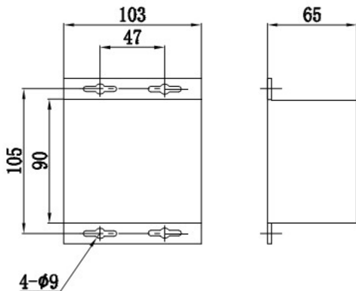
KYXBQ-1000-E尺寸图
