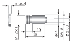
探头
