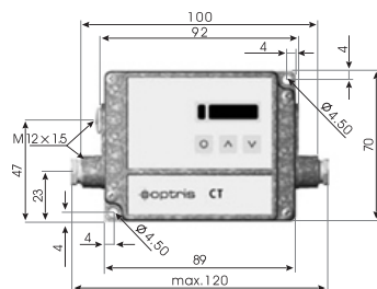
电子盒
