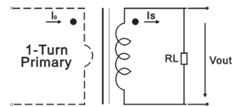
测试电路图 Test Circuit
