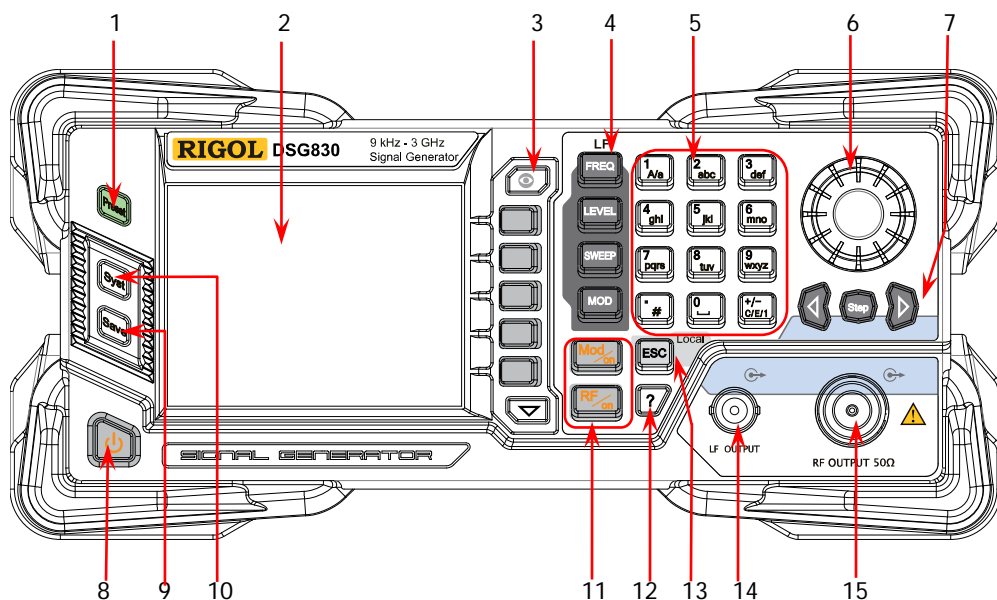
图 1-4 前面板
