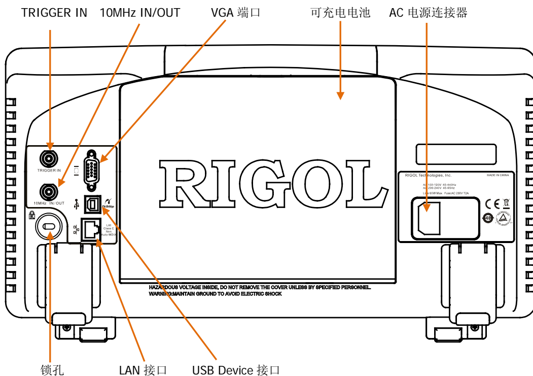
图 1-7 后面板视图
