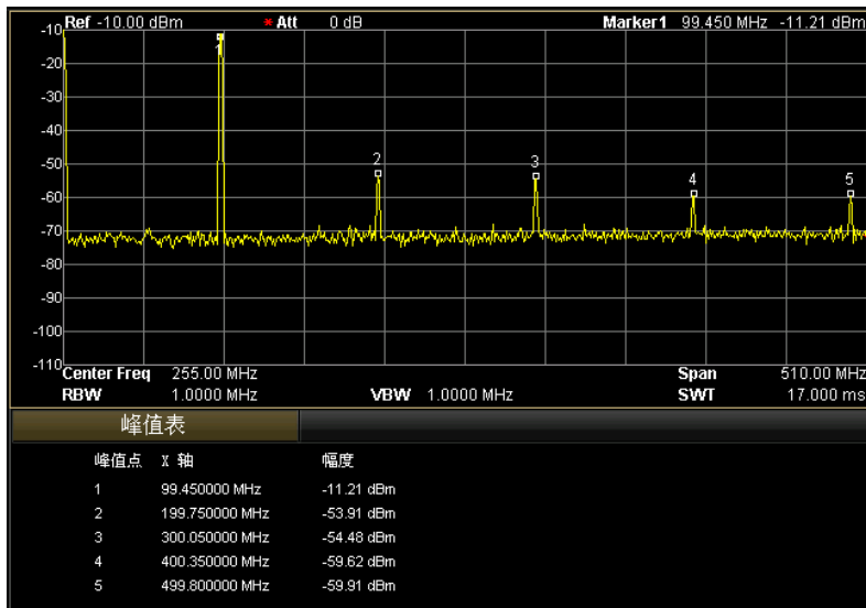
图 2-28 峰值表
