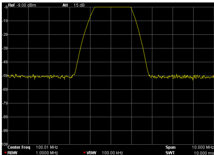
图 2-6 自动量程操作前
