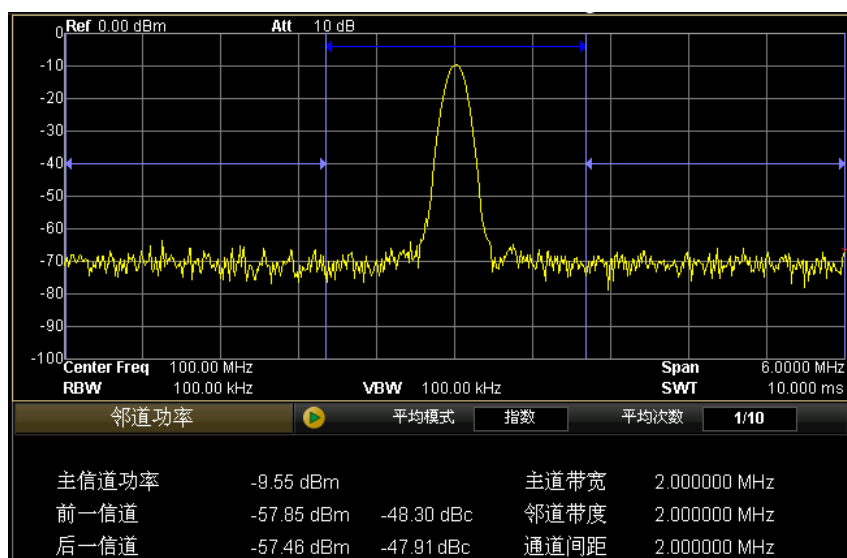
图 3-7 邻道功率测量结果
