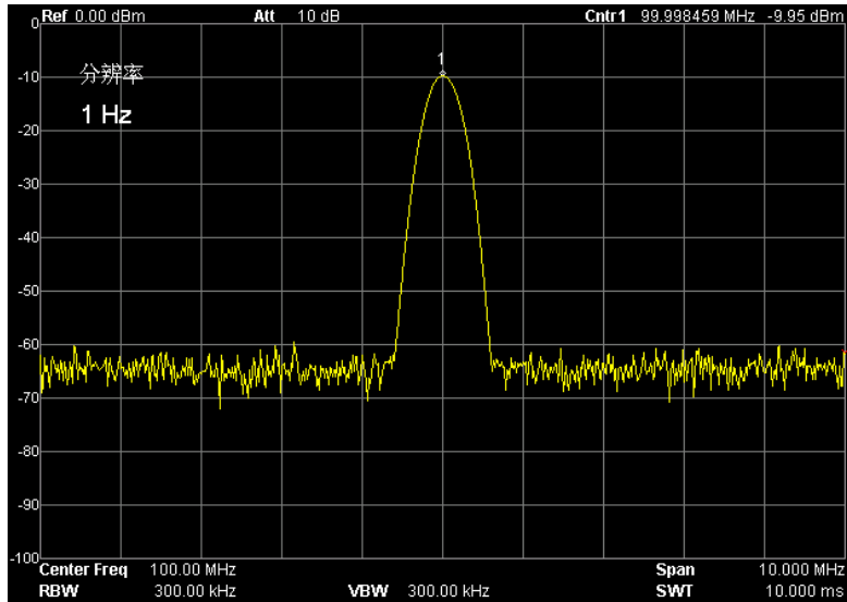
图 3-2 频率测量结果
