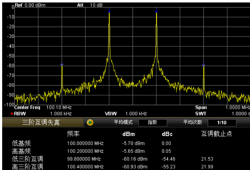
图 3-15 高级功能测量三阶互调失真
