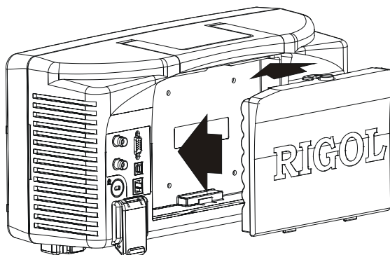
图 1-17 安装电池
