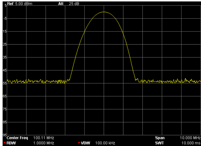
图 2-7 自动量程操作后
