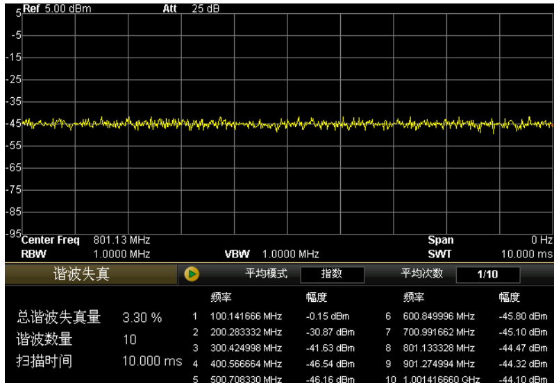
图 2-21 谐波失真测量界面
