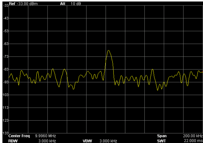
图 2-9 自动搜索信号前
