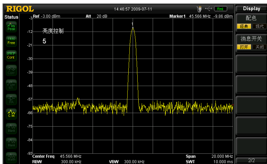
图 2-30 经典显示风格
