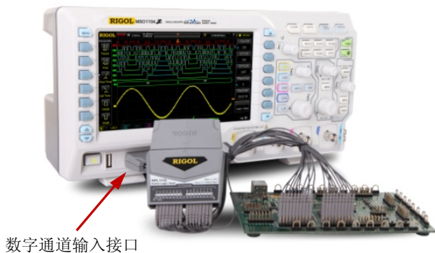
图 1-6 连接逻辑探头
