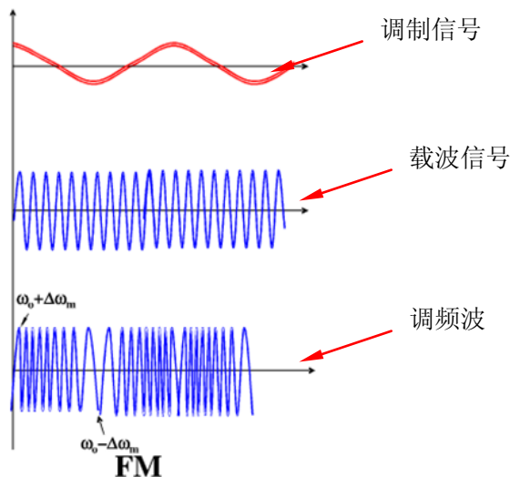
图 13-11 调频
