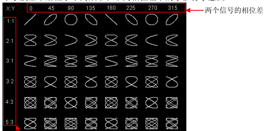
两个信号的频率比
