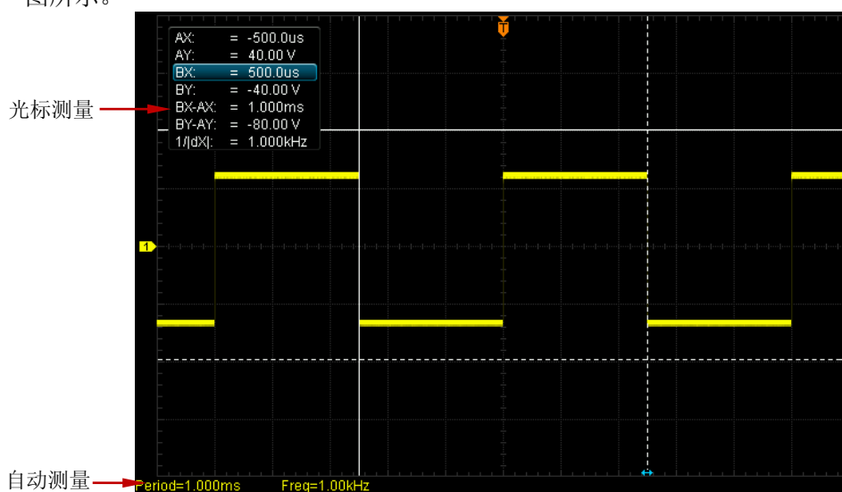
图 6-6 手动光标测量实例
