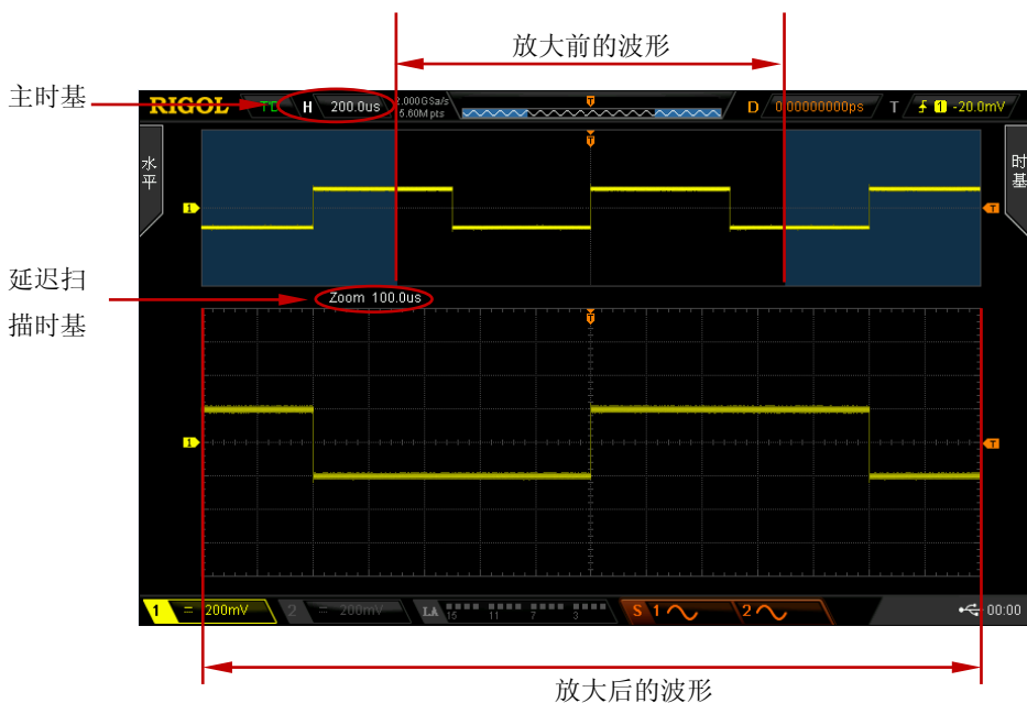
图 3-1 延迟扫描模式
