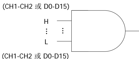
图 5-8 码型触发
