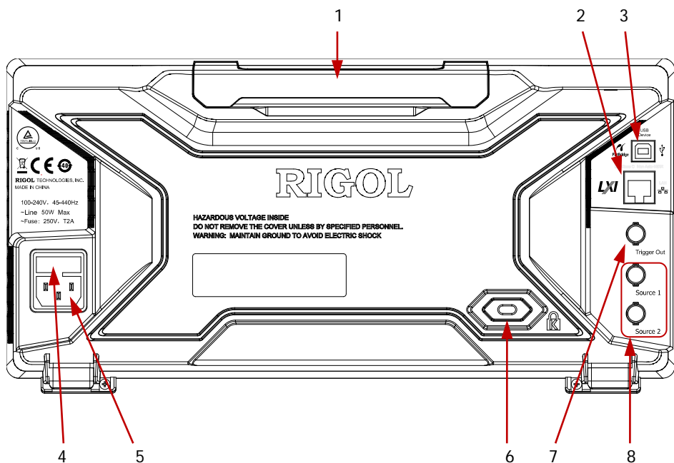
图 1-11 后面板总览
