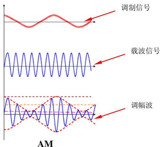
图 13-9 调幅
