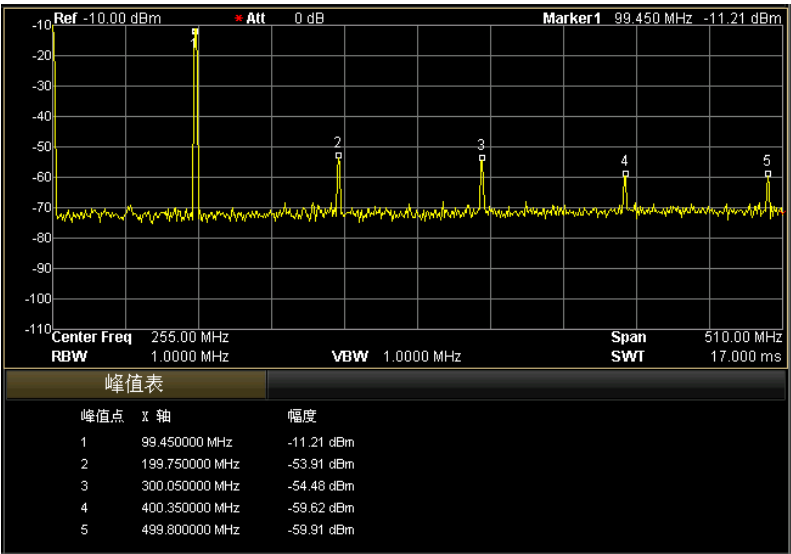
图 2-28 峰值表
