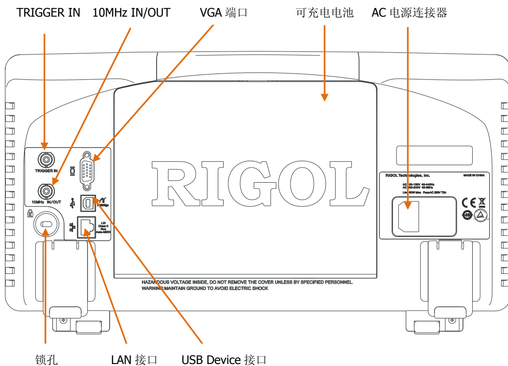
图 1-7 后面板视图
