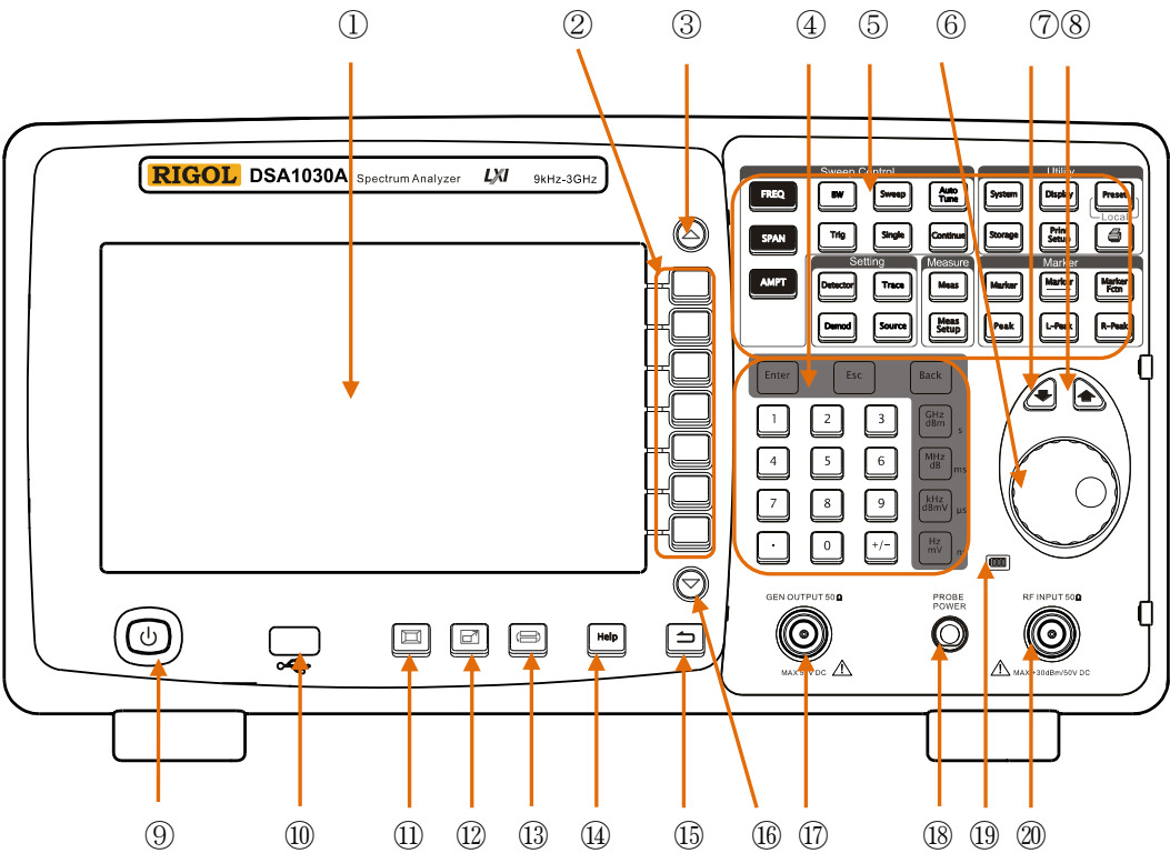
图 1-1 前面板视图
