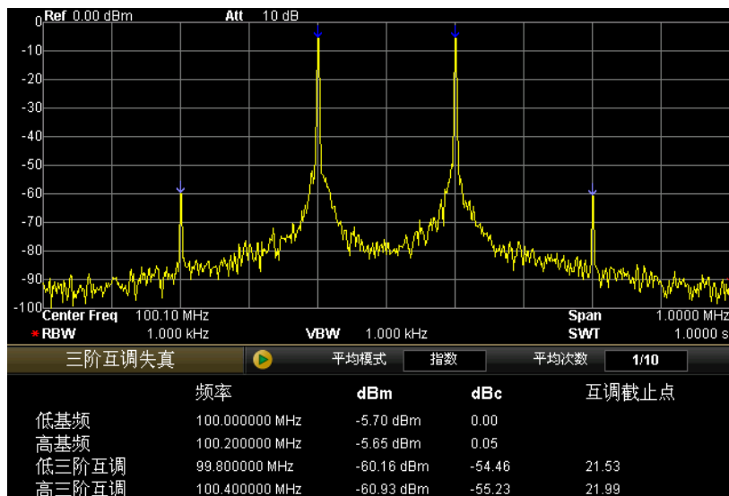
图 2-22 三阶互调失真测量界面
