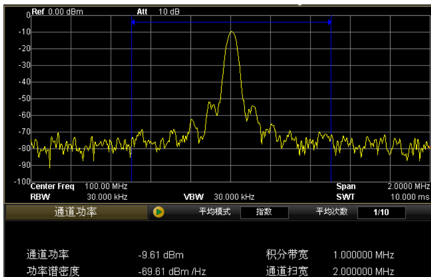
图 3-8 通道功率测量结果
