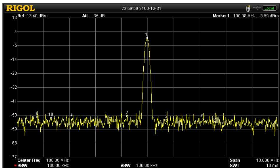
图 2-34 全屏显示
