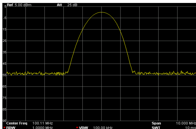
图 2-7 自动量程操作后
