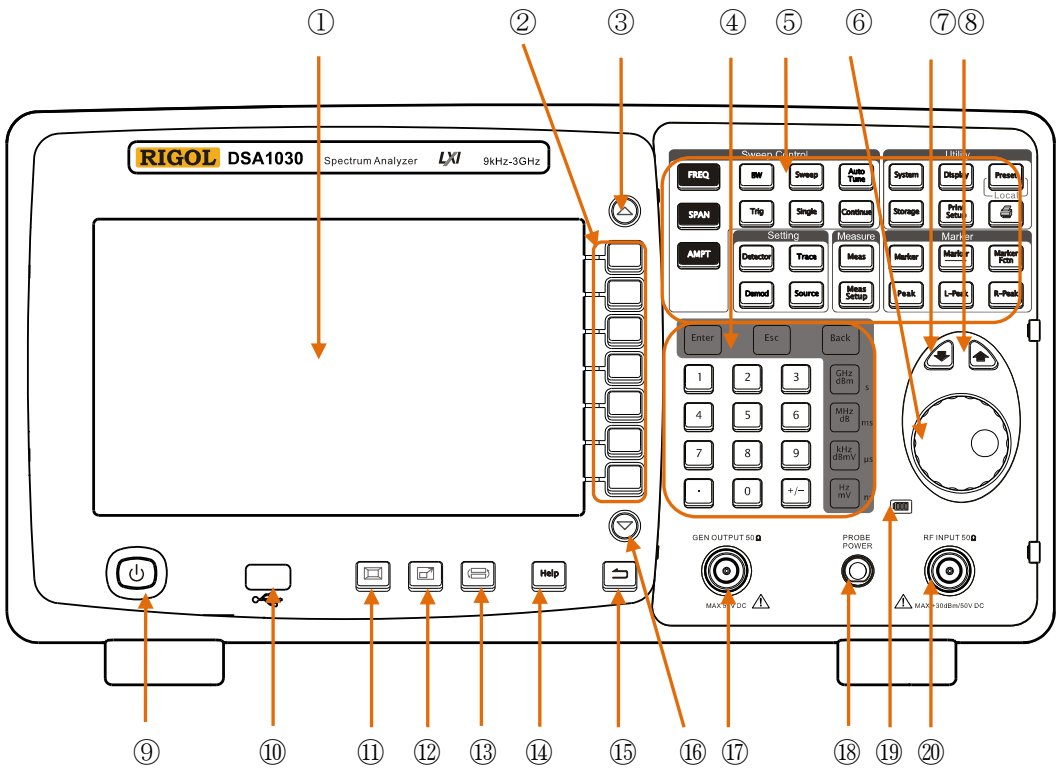
图 1-1 前面板视图
