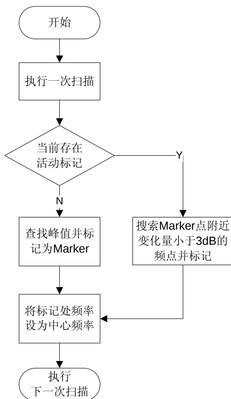
图 2-1 信号追踪过程
