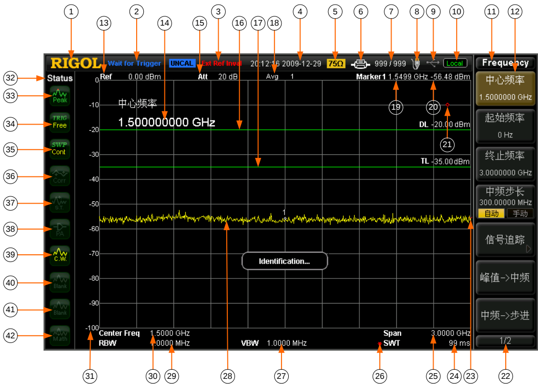
图 1-20 用户界面
