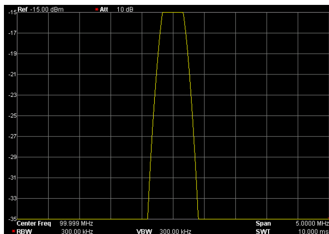
图 2-4 自动定标操作前
