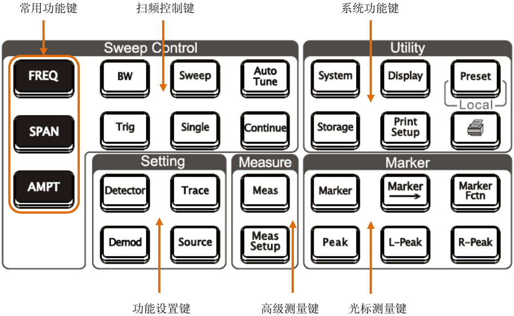
图 1-2 功能键示意图
