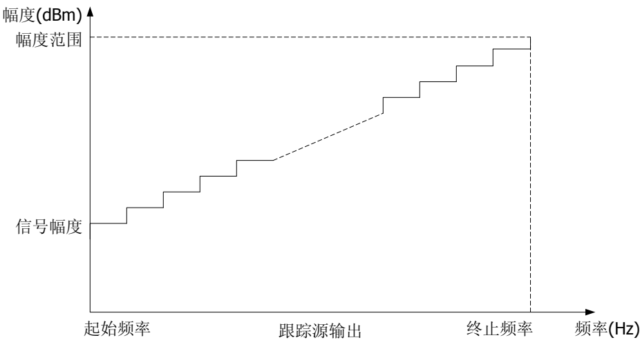
图 2-14 功率扫描示意图
