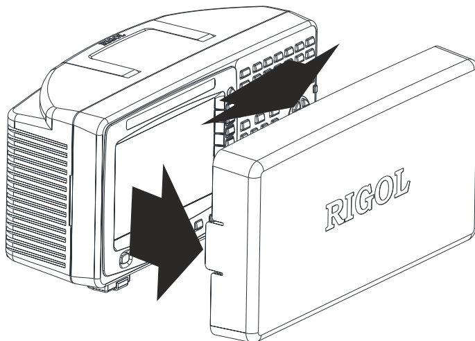
图 1-14 拆卸前面板保护壳
