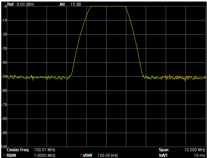
图 2-6 自动量程操作前
