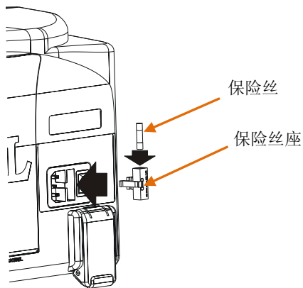
图 1-19 更换保险丝
