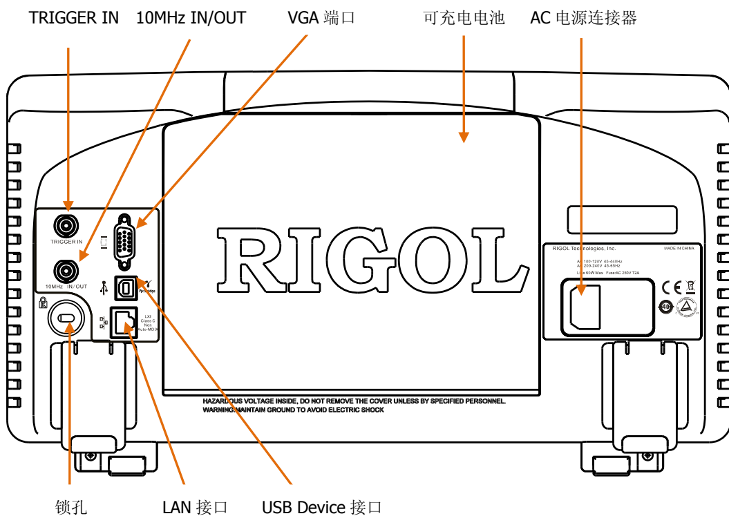
图 1-7 后面板视图
