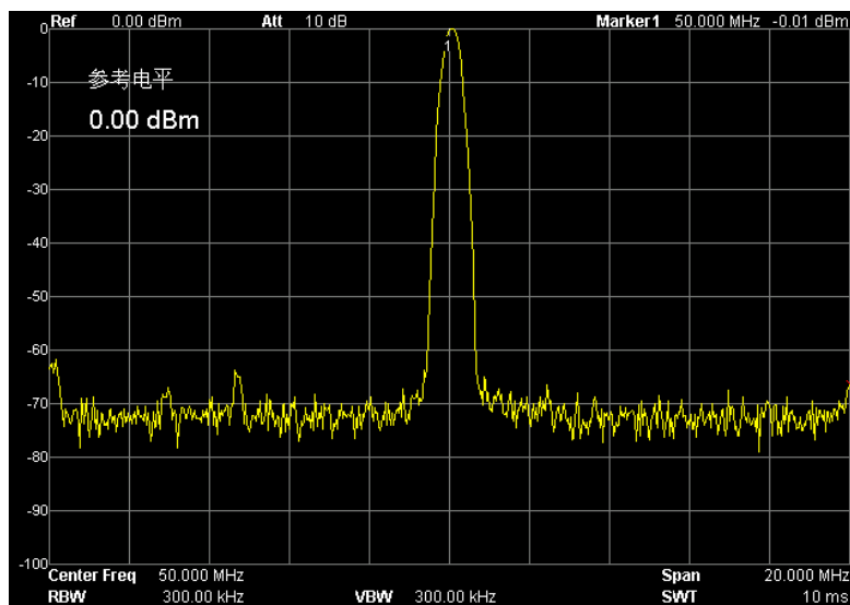
图 1-24 测量结果
