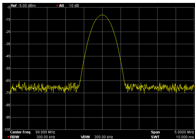
图 2-5 自动定标操作后
