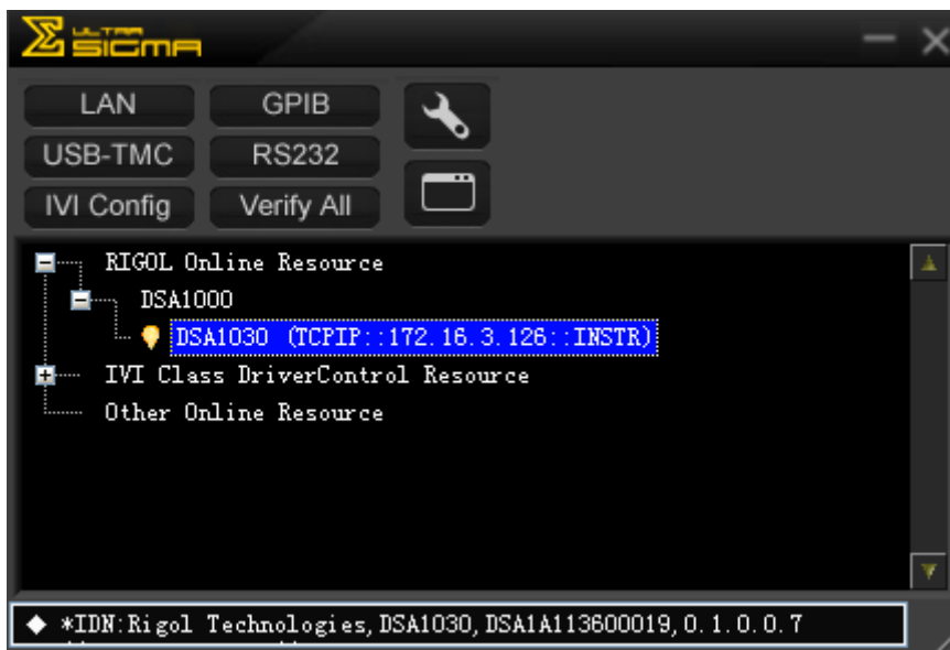
图 4-5 查看网络资源
