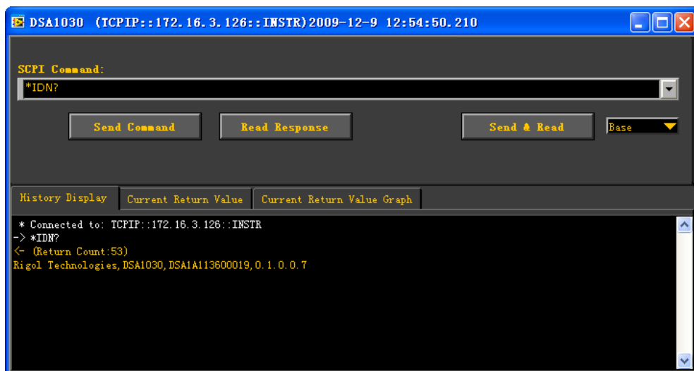
图 4-6 通过 LAN 读写命令
