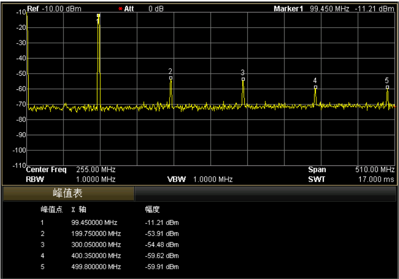
图 2-28 峰值表
