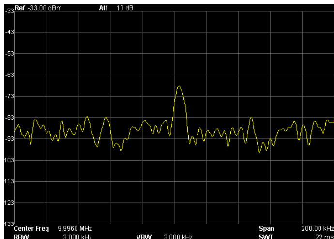
图 2-9 自动搜索信号前
