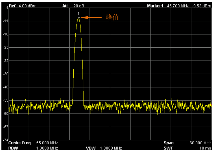
图 2-2 峰值->中频操作前
