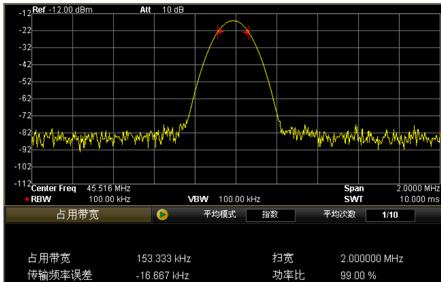
图 2-18 占用带宽测量界面
