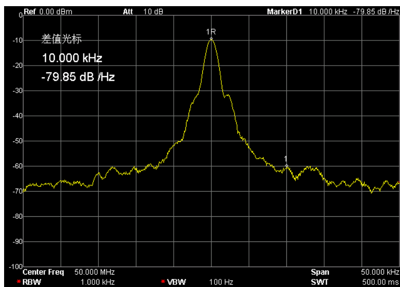
图 3-4 相位噪声测量结果
