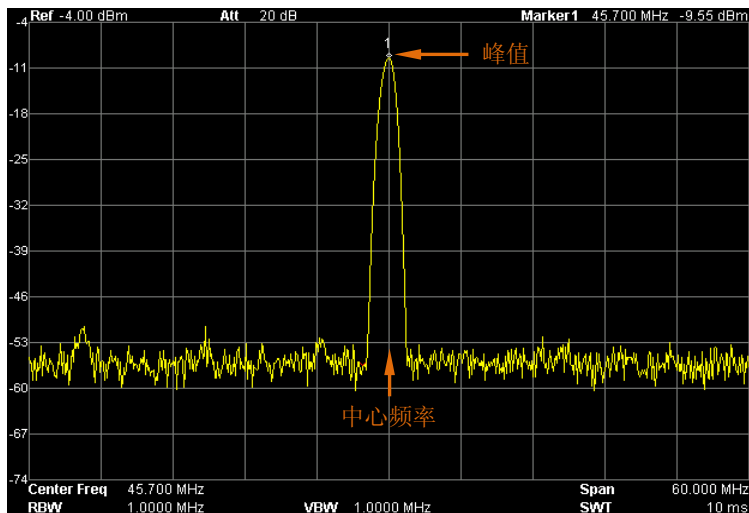
图 2-3 峰值-&gt;中频操作后
