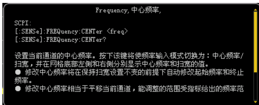
图 1-25 帮助界面
