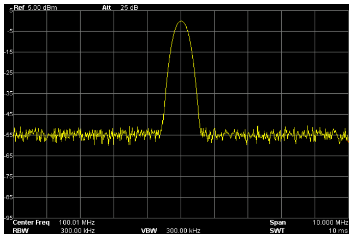
图 2-10 自动搜索信号后
