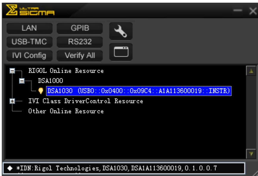
图 4-2 查看 USB 设备资源
