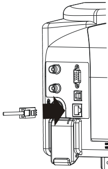
图 1-13 LAN 接口连接
