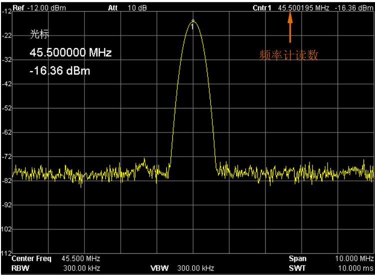
图 2-27 频率计测量
