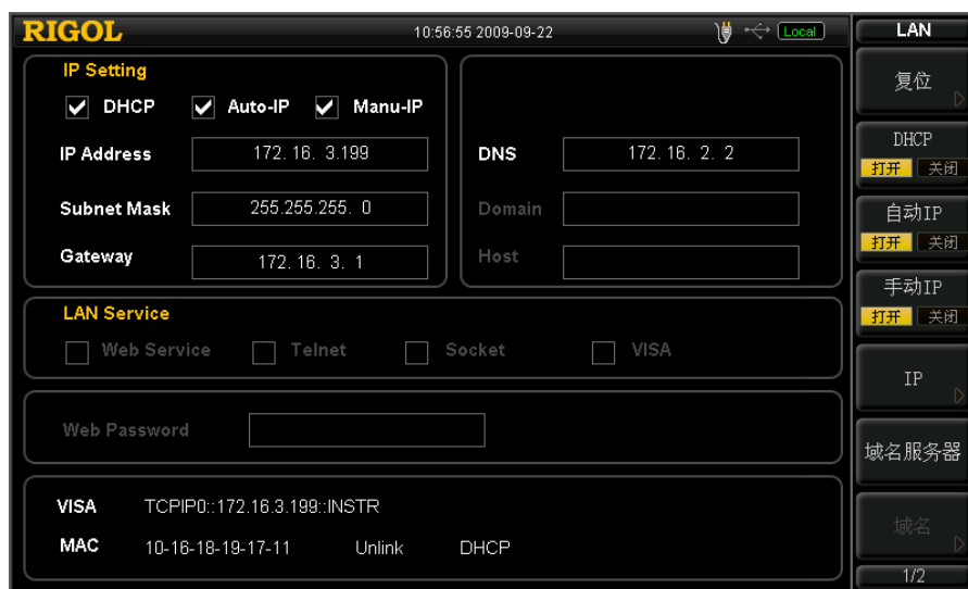
图 2-29 LAN 参数设置
