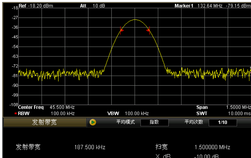
图 2-19 发射带宽测量界面
