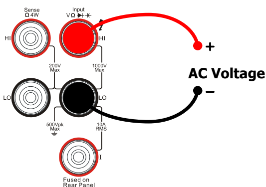
图 2-8 交流电压测量连接示意图
