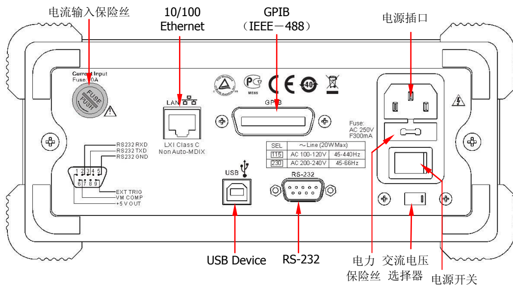
图 1-4 DM3058 后面板示意图
