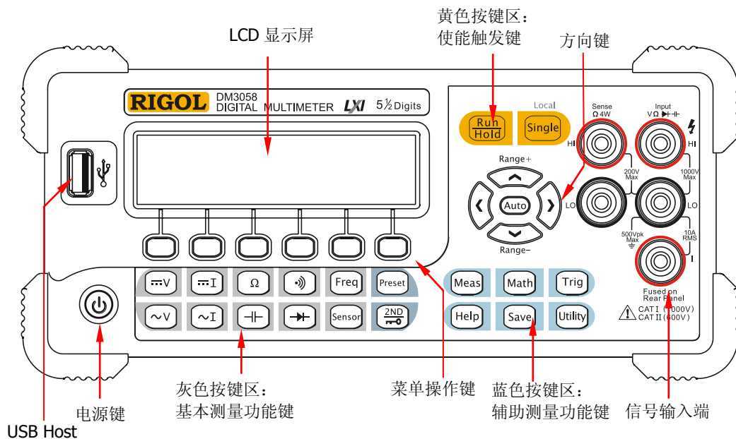
图 1-3 DM3058 前面板示意图
