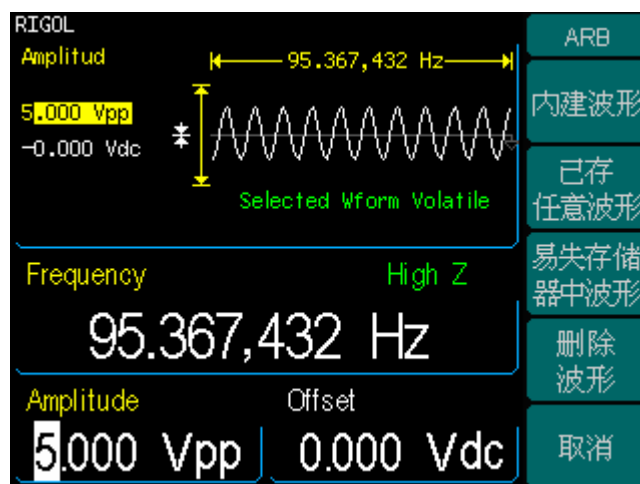
图 2—52 编辑波形界面
