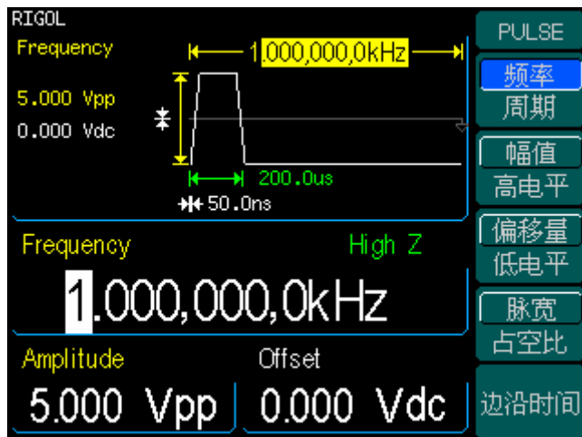
图 1—11 脉冲波图形界面
