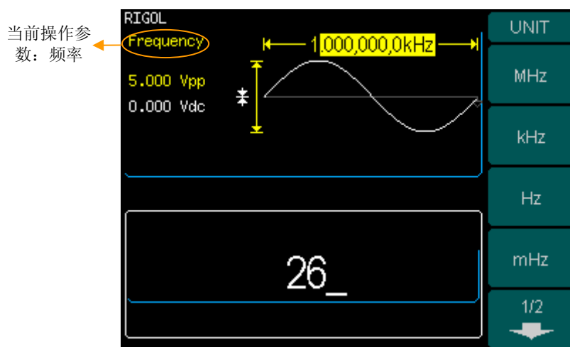
图 2—3 设置频率的参数值
