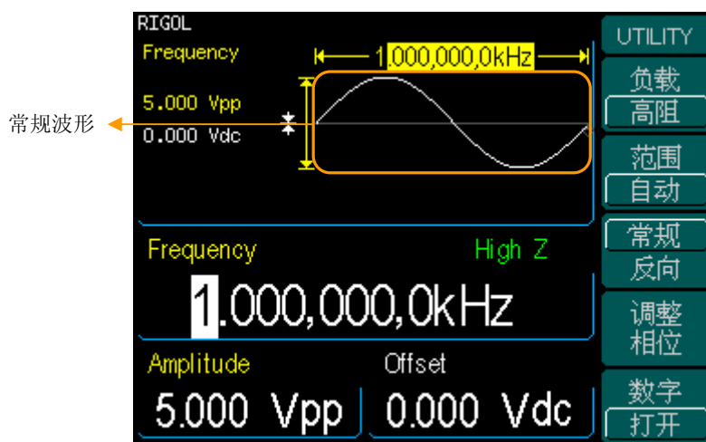
图 2—65 常规波形
