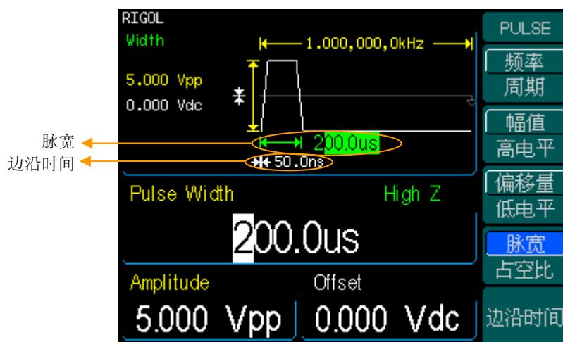
图 2—12 脉冲波形及参数值显示窗口
