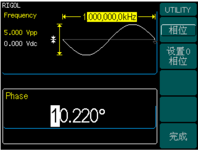
图 2—67 相位调整设置
