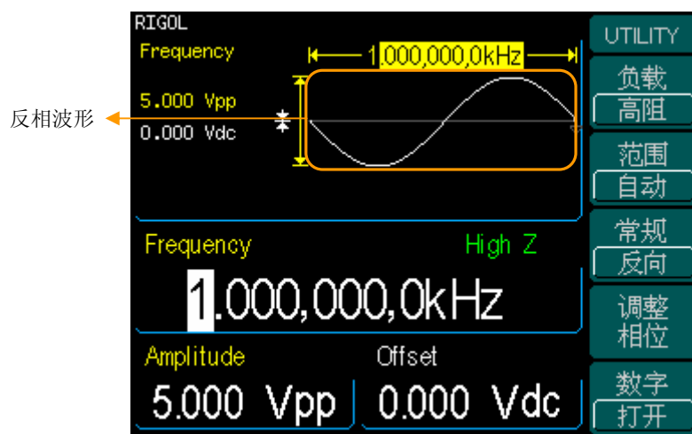
图 2—66 反向波形
