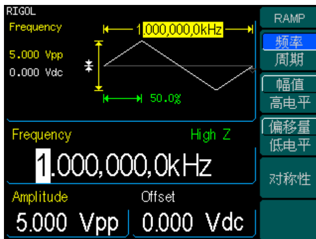
图 1—10 锯齿波显示界面
