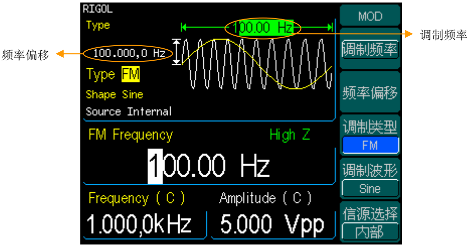
图 2－32 频率调制波形及参数显示窗口
