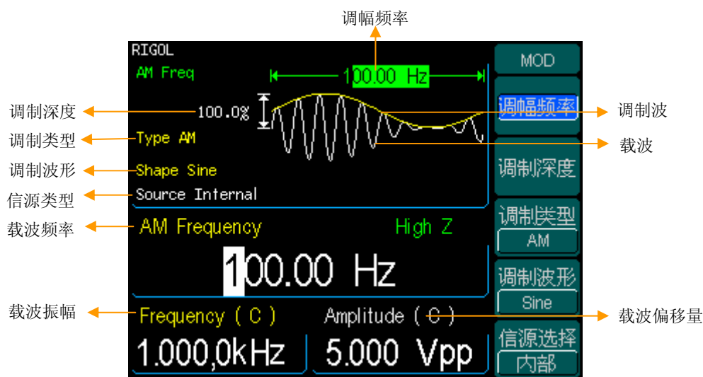
图 2—30 调制波形及参数值显示窗口
