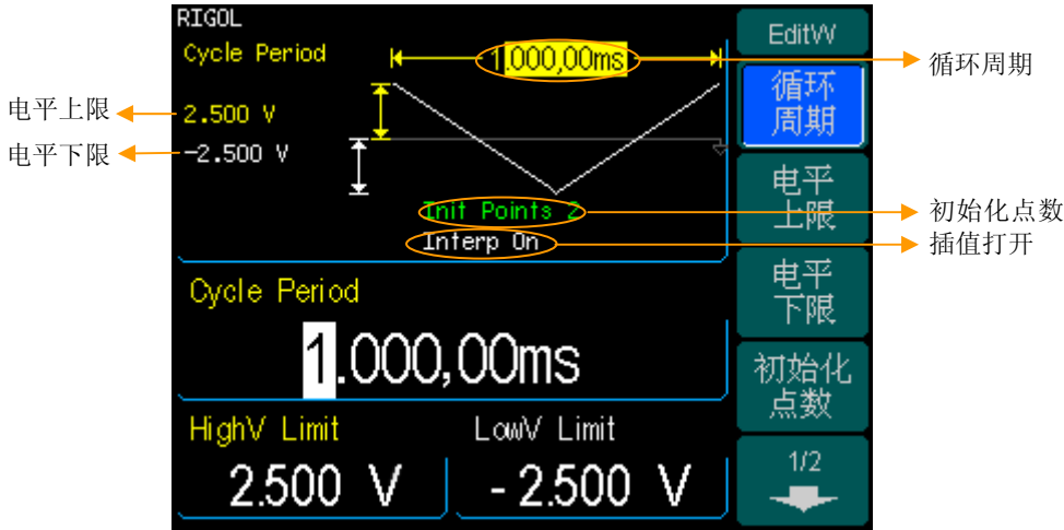
图 2—25 创建新波形的参数设置界面
