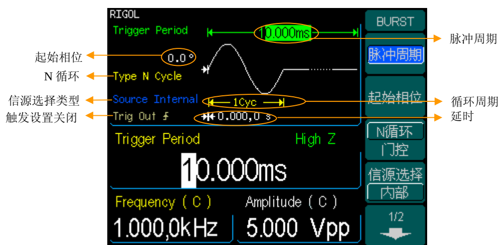
图 2-42 脉冲串波形及参数值显示窗口
