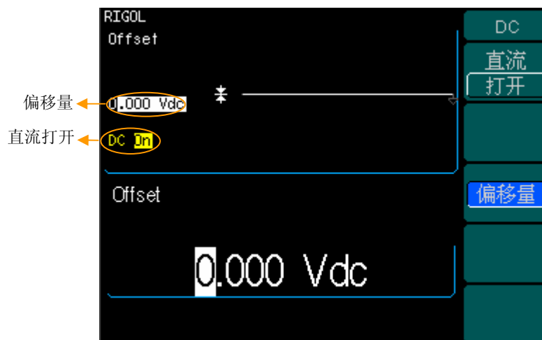
图 2—62 设置直流输出
