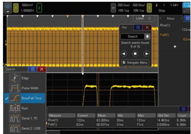
图10: 4000 X系列能够使用不同的上升沿捕获数据信号。使用搜索和导航功能，示波器能够查找、标记(白色三角形)和快速导航到16个出现“不符合一致性的”上升沿的位置。
