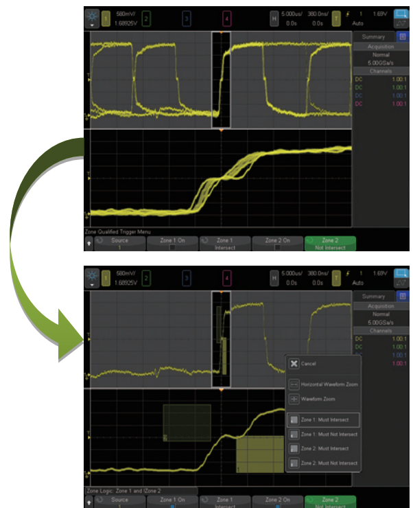
图 16. 隔离感兴趣的信号前所未有的容易。
