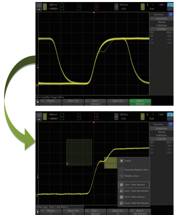
图 15. 当您看到信号异常时，您要做的就是绘制一个区域方框，以便在这些异常信号上进行触发。
