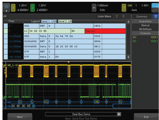
图 19: 双路串行总线 CAN 和 LIN 解码和交叉“列表”显示。
