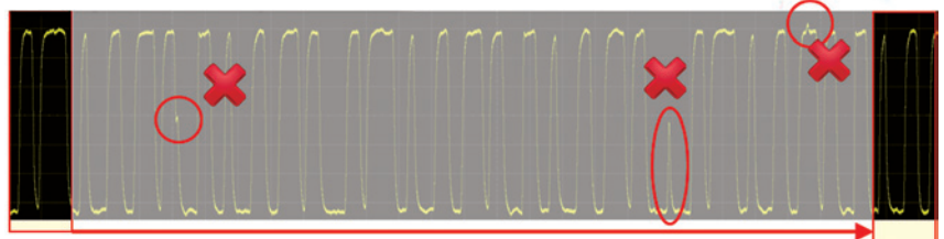
图4: 其它厂商的具有50000个波形/秒更新率的示波器。长静寂时间会减少捕获罕见事件的几率。
