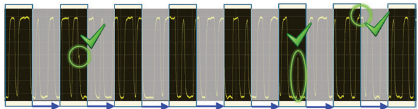
图5: 具有1000000个波形/秒更新率的InfiniiVision 4000 X系列。短静寂时间可增加捕获罕见事件的几率。
