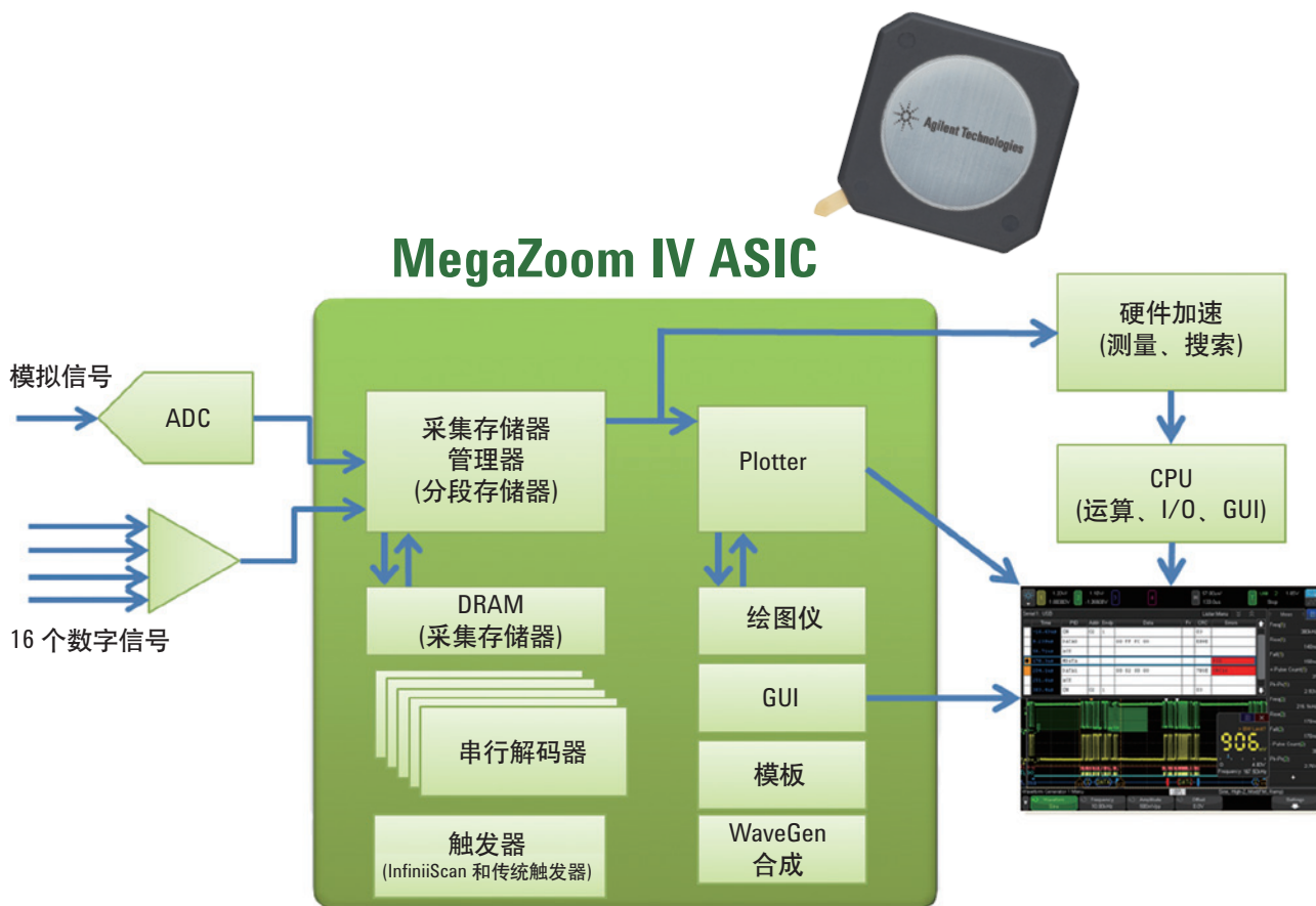
图6. MegaZoom IV 智能存储器 ASIC 使 4000 X 系列示波器的响应性、速度和波形更新率不受任何影响。核心波形运算无需依靠 CPU 进行。
