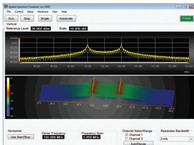
图 39: ASV 频谱图测量串接显示视图。
