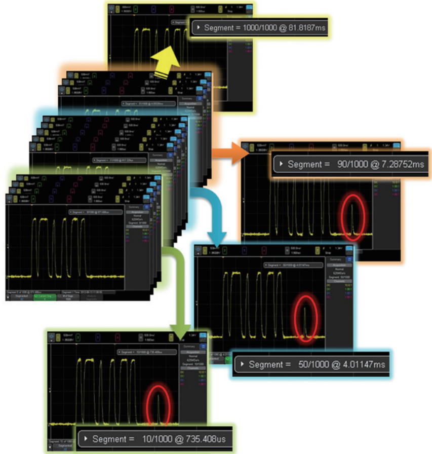
图7: 分段存储器能够高效地对存储器进行管理,捕获多达1000个您感兴趣的分段,因此是能够轻松捕获偶发事件和异常事件的高效率、超深度存储器示波器。
