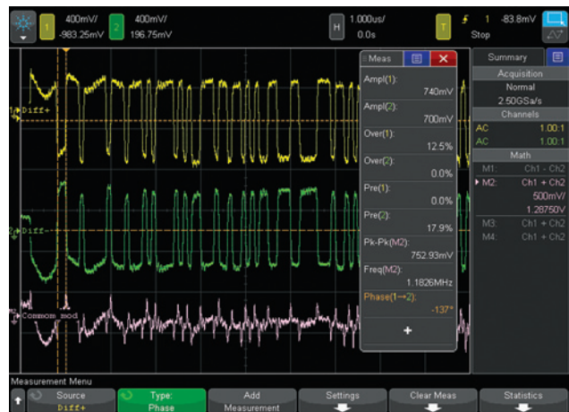
图 23: 差分任意波形信号的双通道 WaveGen 输出。共模作为运算函数显示。
