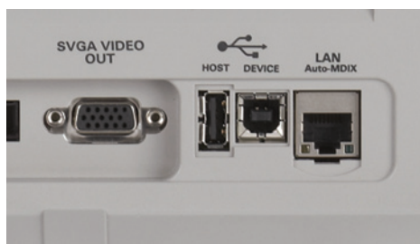
图 35: 标配的 VGA 输出、USB 主机和设备以及 LAN 接口。
