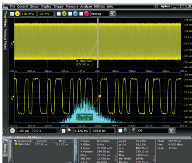
图 38: InfiniiView 能够进行各种先进的信号分析，同时还能提供广泛而直观的波形文档。
