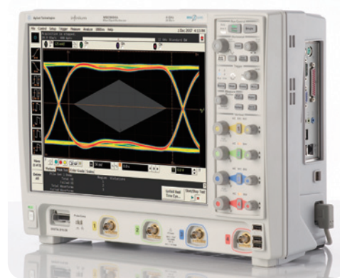
图 2: InfiniiVision 9000 系列示波器。
