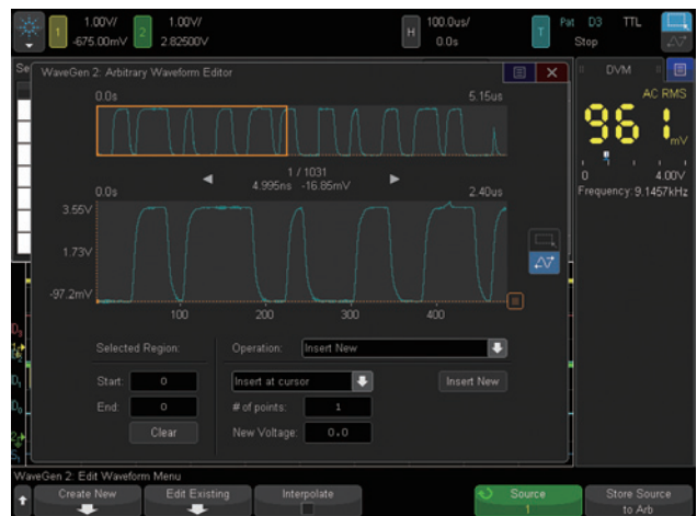
图 22: WaveGen 任意波形编辑屏幕。
