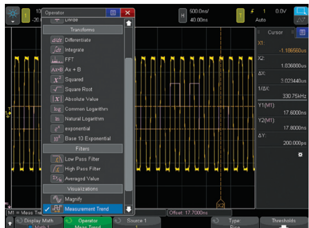
图 29: 4000 X 系列作为标准配置提供各种先进的运算函数。
