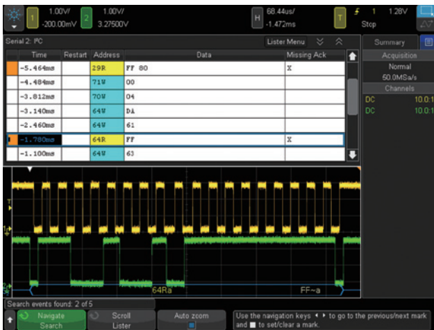
图11: 使用误码条件搜索，4000 X系列可以在I 2 C串行总线中快速找到5处具有丢失确认信息的结果。导航特性使您可以在误码间移动，并自动进行缩放以显示误码数据包。
