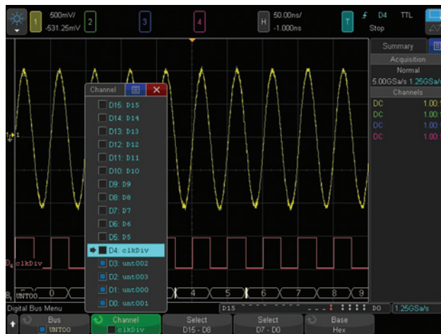
图27. FPGA 动态探头路由由内部 FPGA 信号, 该信号由 4000 X 系列进行捕获, 与设计中的这个外部模拟正弦波进行关联。
