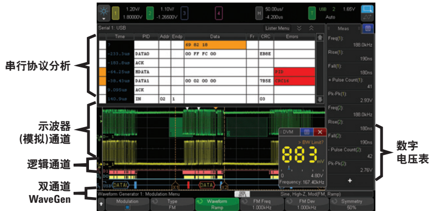
图 17: 4000 X 系列将 5 种仪器的功能完美集成到一起。
